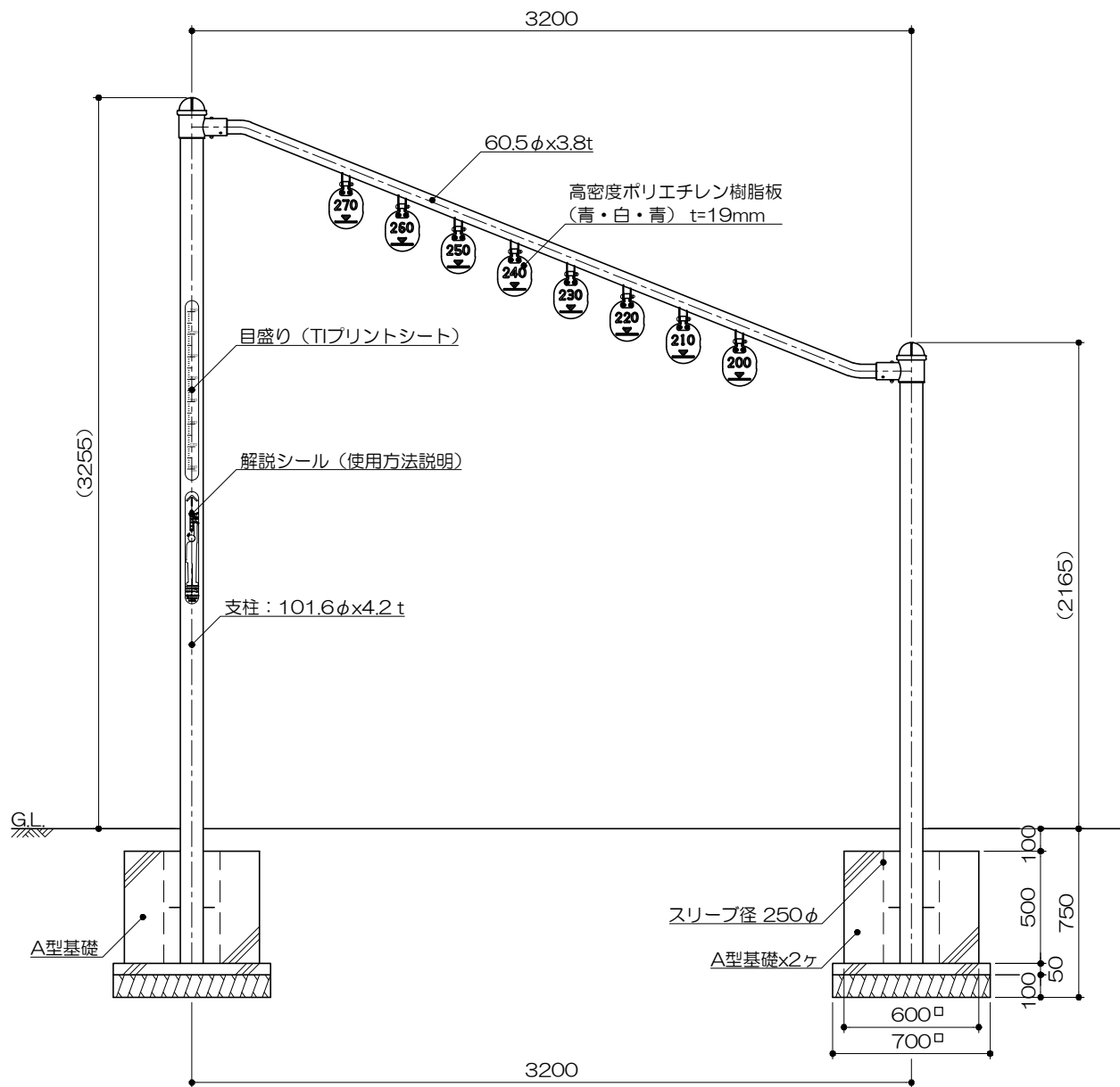
立面図 S= 1 : 30
