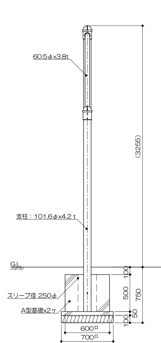
側面図 S= 1 : 30
