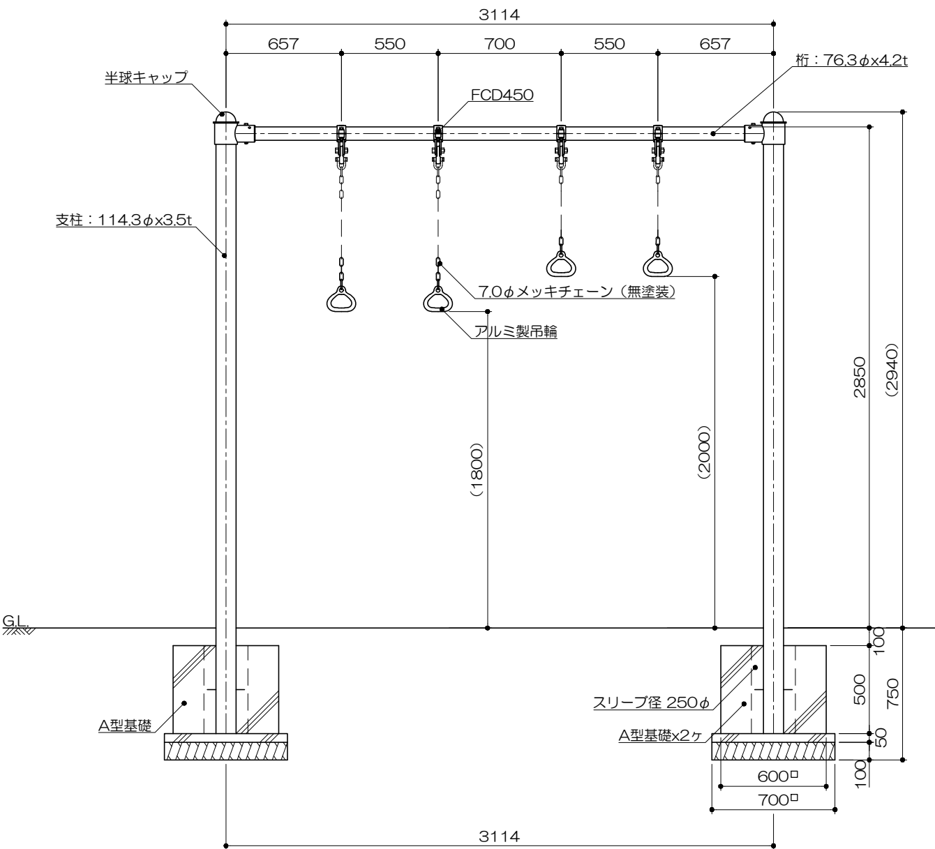
立面図 S= 1 : 30
