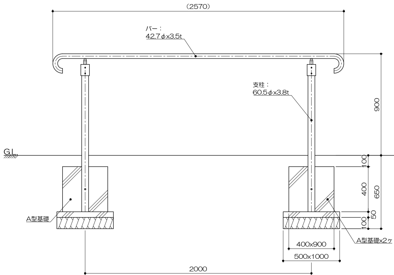
立面図 S= 1 : 20
