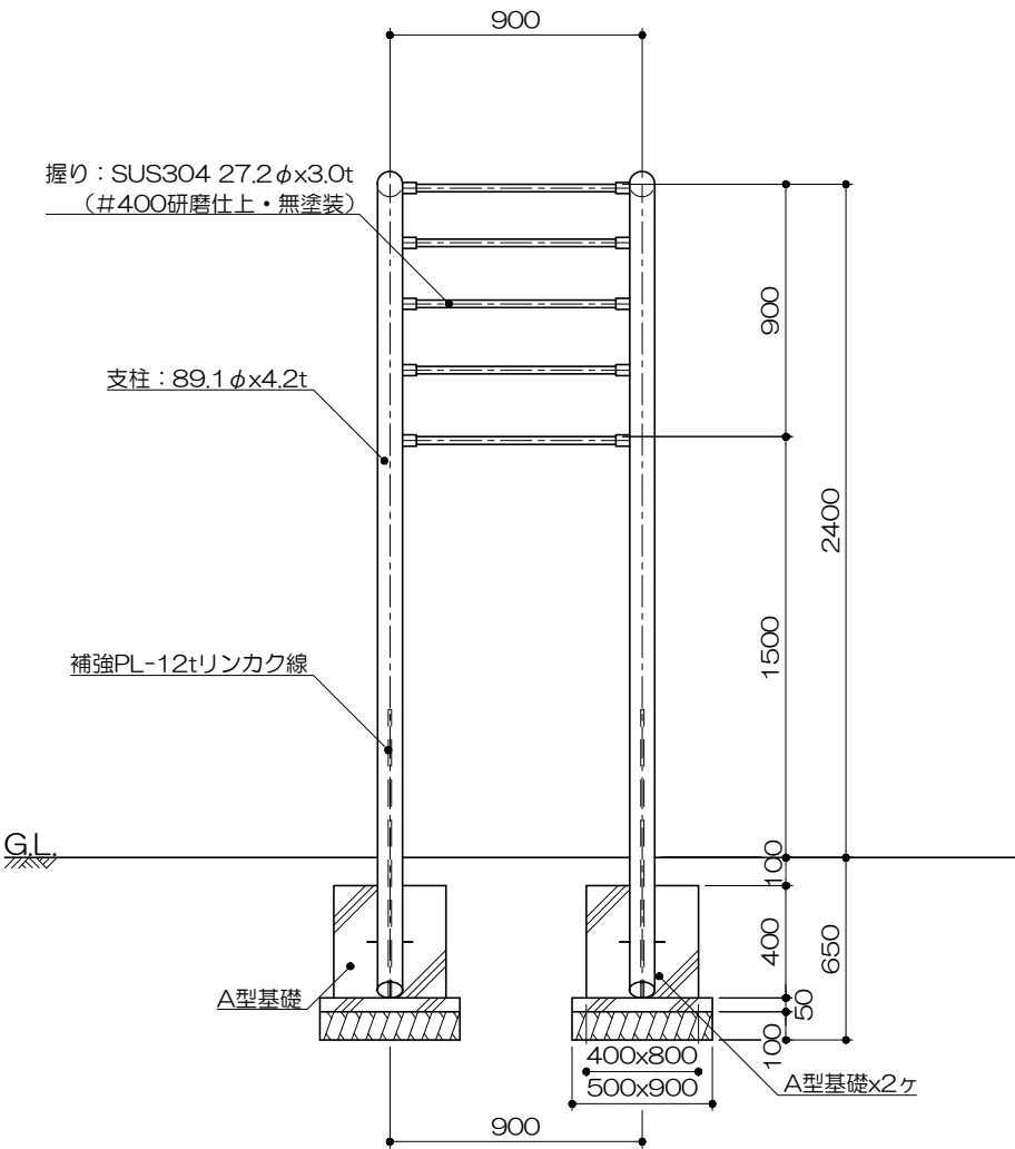
立面図 S= 1 : 30
