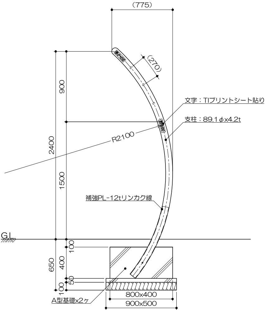
側面図 S= 1 : 30
