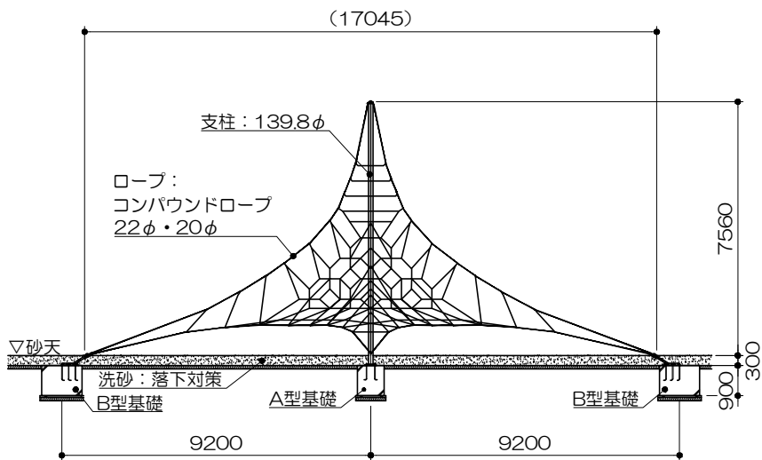
立面図 S= 1 : 200
