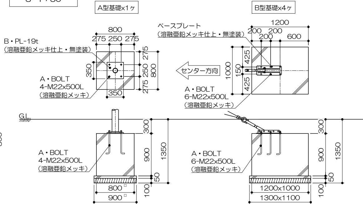
基礎リスト S= 1 : 50
