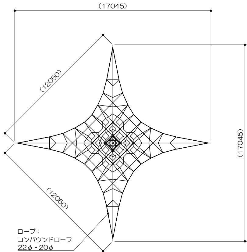
平面図 S= 1 : 200
