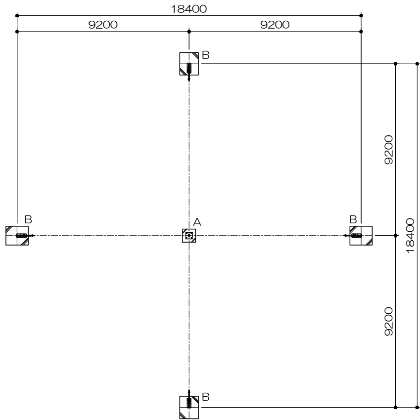
基礎平面図 S= 1 : 200
