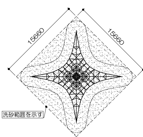
洗砂範囲 S= 1 : 400
