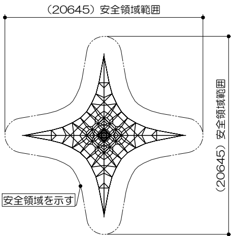
安全領域範囲 S= 1 : 400
