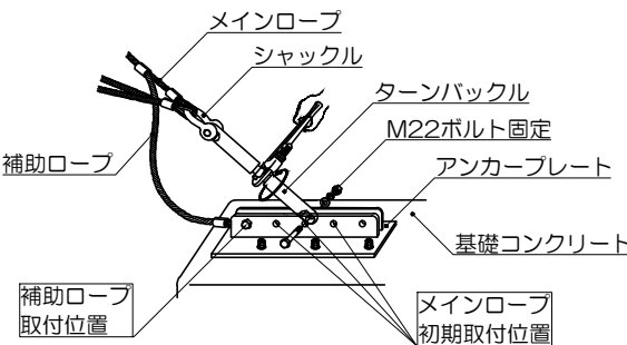
ロープ接続部詳細図
