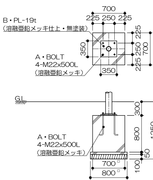
基礎リスト S= 1 : 50
