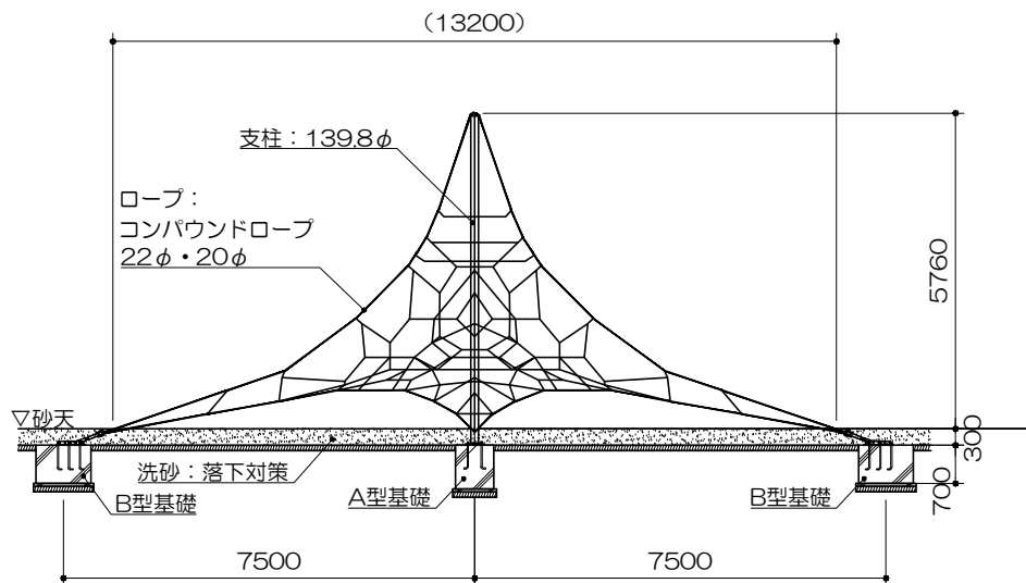
立面図 S= 1 : 150
