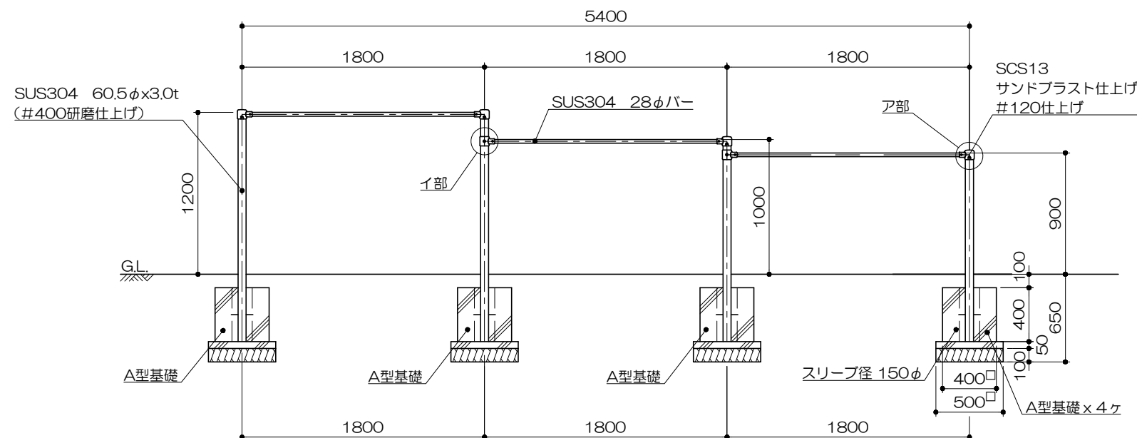
立面図 S= 1 : 40
