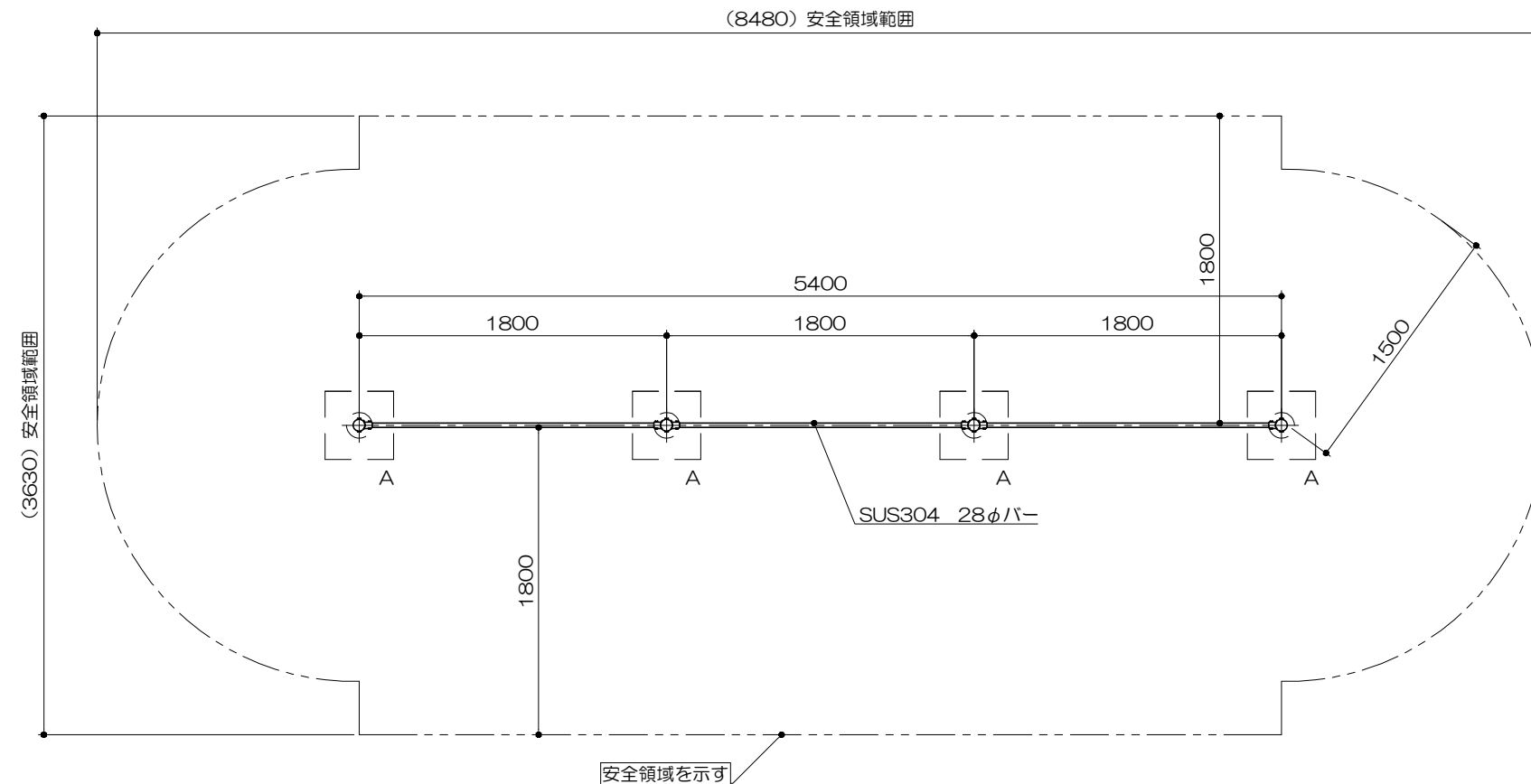
平面図 S= 1 : 40
