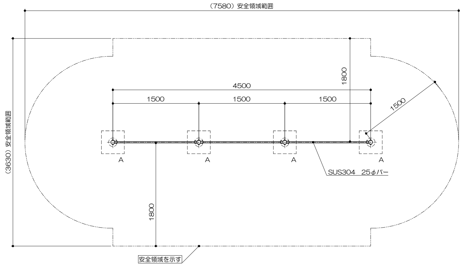
平面図 S= 1 : 40
