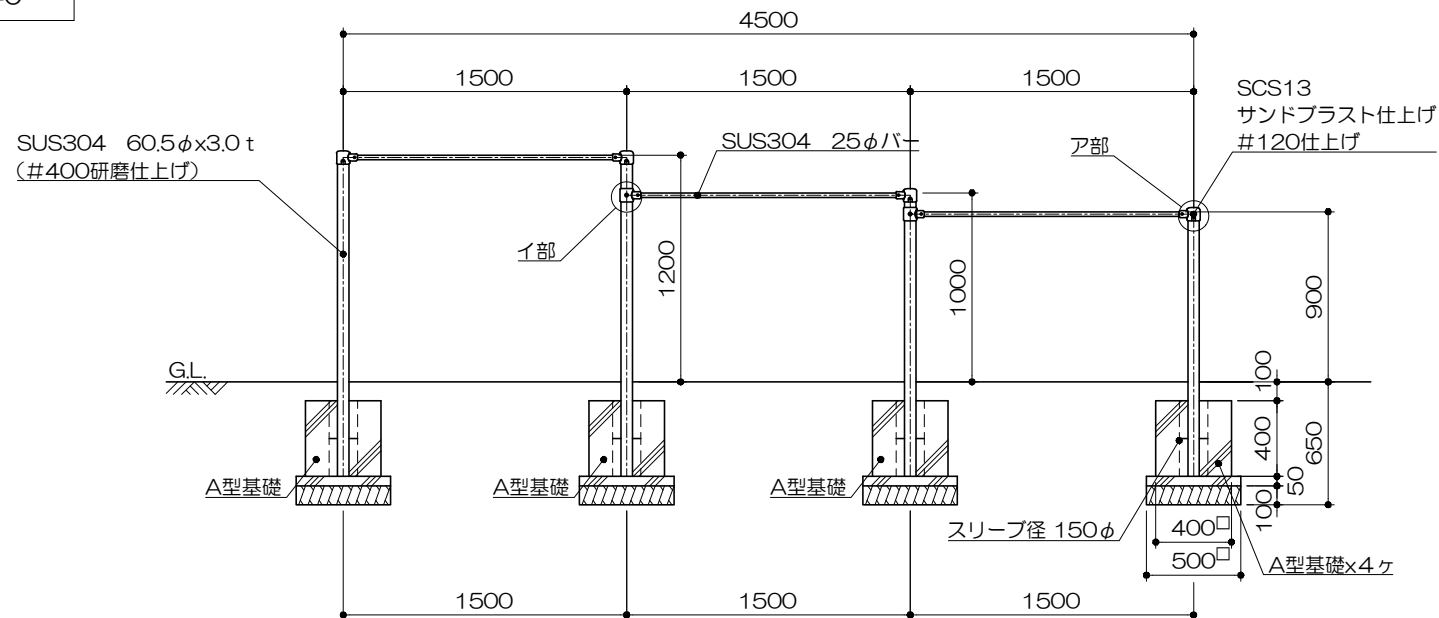
立面図 S= 1 : 40
