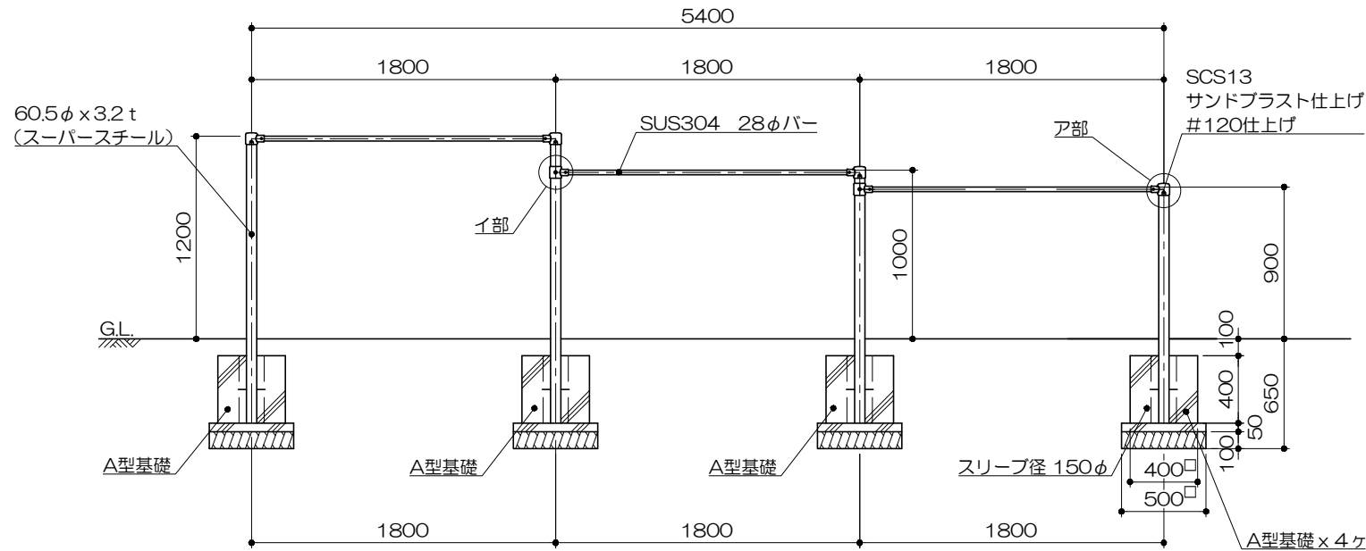
立面図 S= 1 : 40
