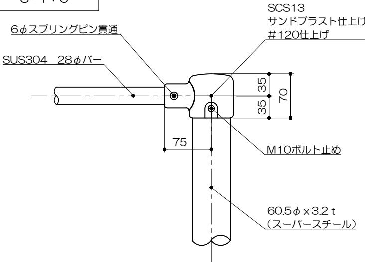
イ部詳細図 S= 1 : 6
