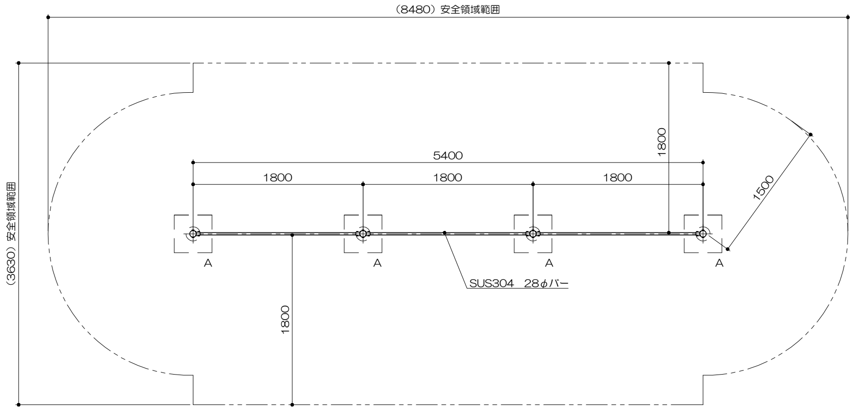
平面図 S= 1 : 40
