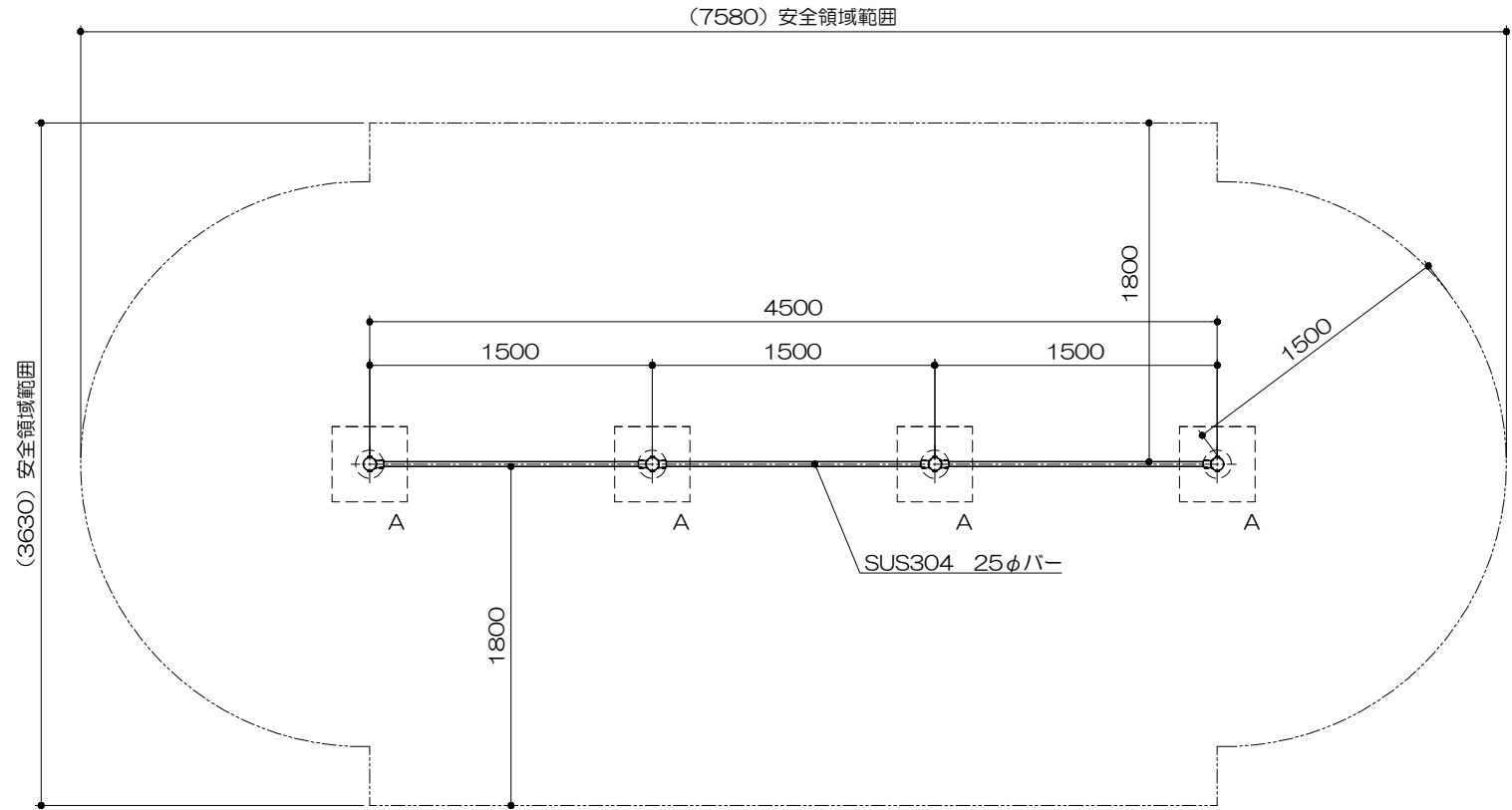
平面図 S= 1 : 40
