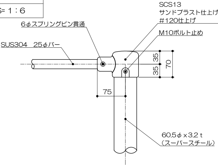
イ部詳細図 S= 1 : 6
