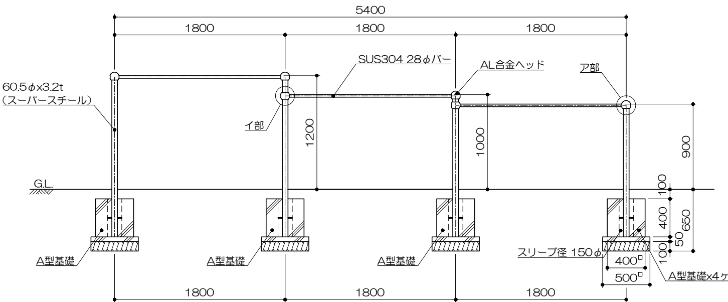
立面図 S= 1 : 40
