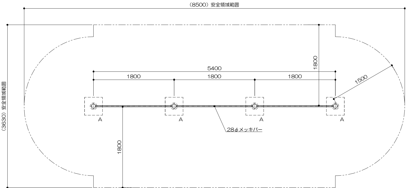
平面図 S= 1 : 40
