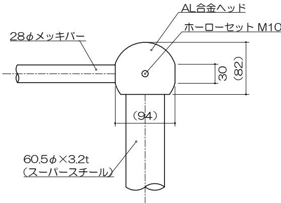
ア部詳細図 S= 1 : 6
