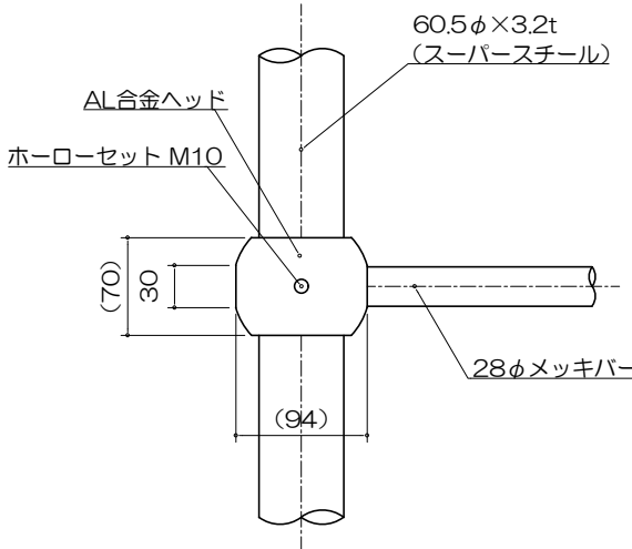
イ部詳細図 S= 1 : 6
