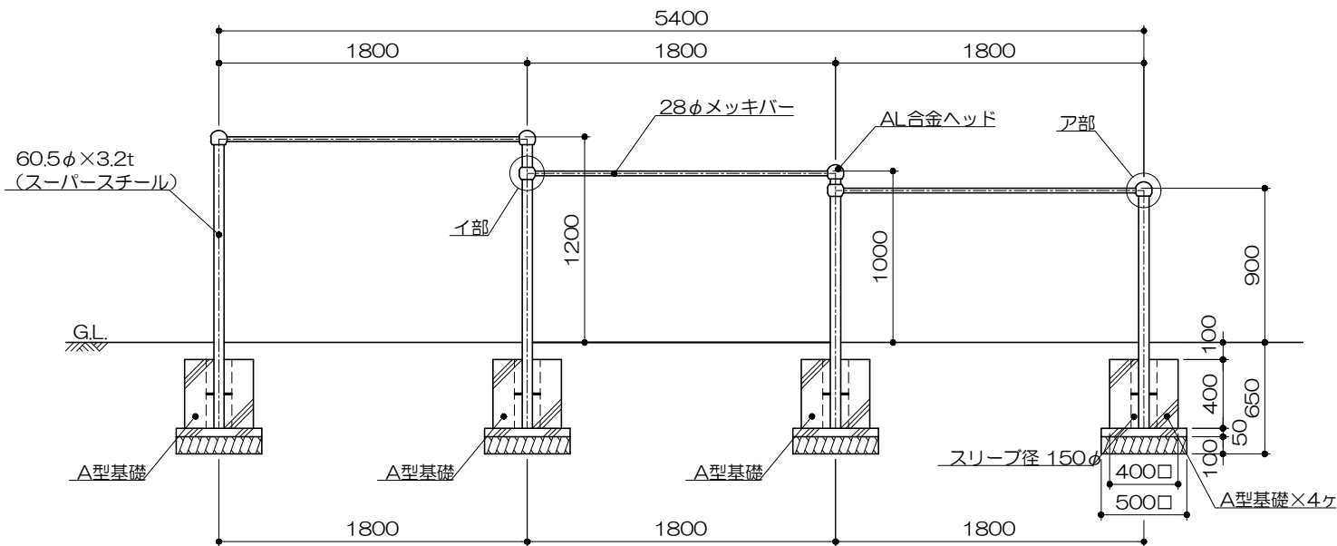
立面図 S= 1 : 40
