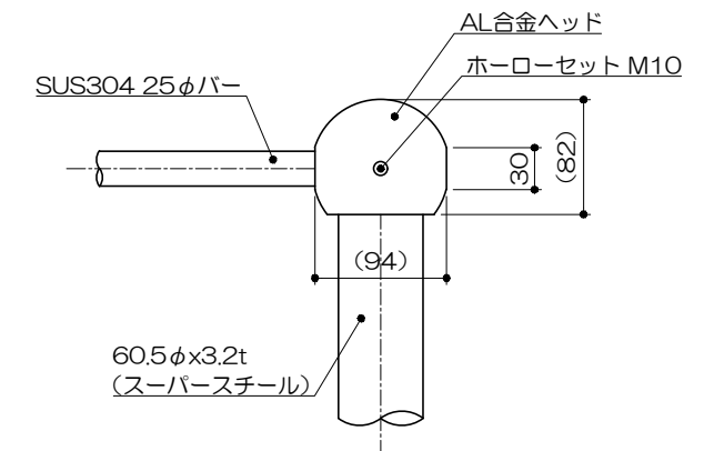
イ部詳細図
