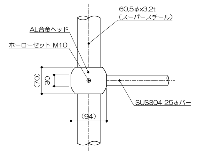
イ部詳細図
