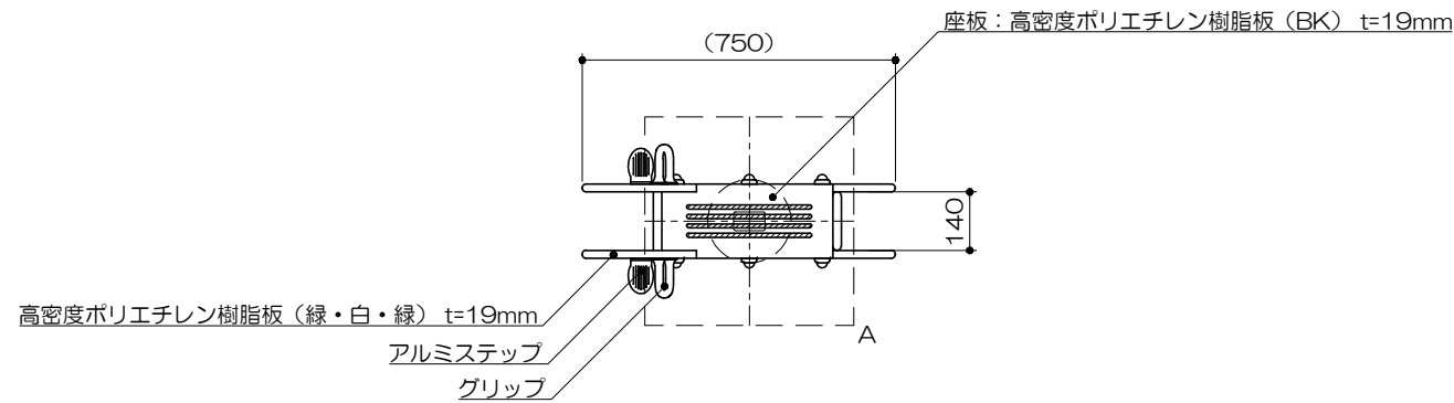
平面図 S= 1 : 20
