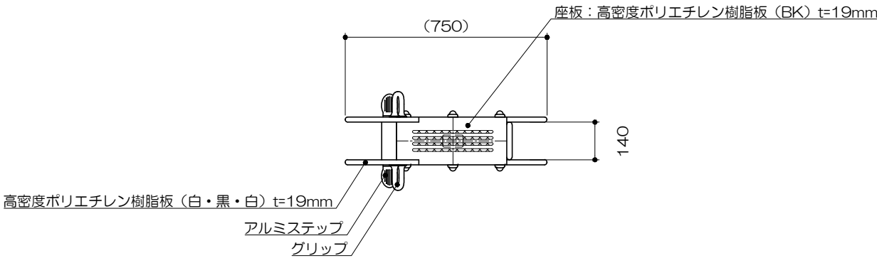
平面図 S= 1 : 20
