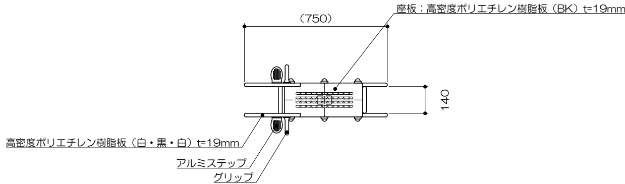
平面図 S= 1 : 20
