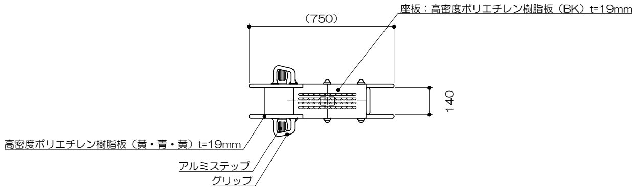
平面図 S= 1 : 20
