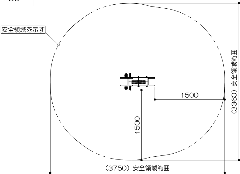
安全領域範囲 S= 1 : 50
