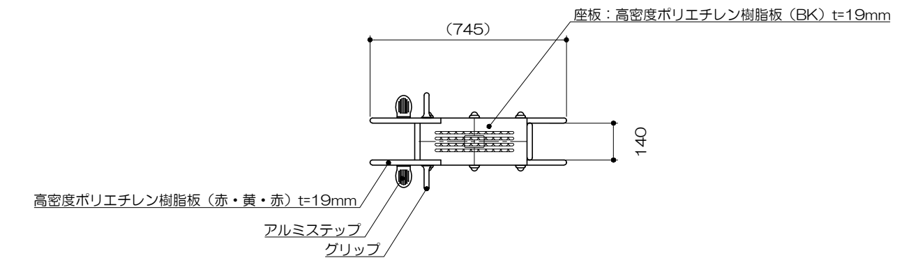
平面図 S= 1 : 20
