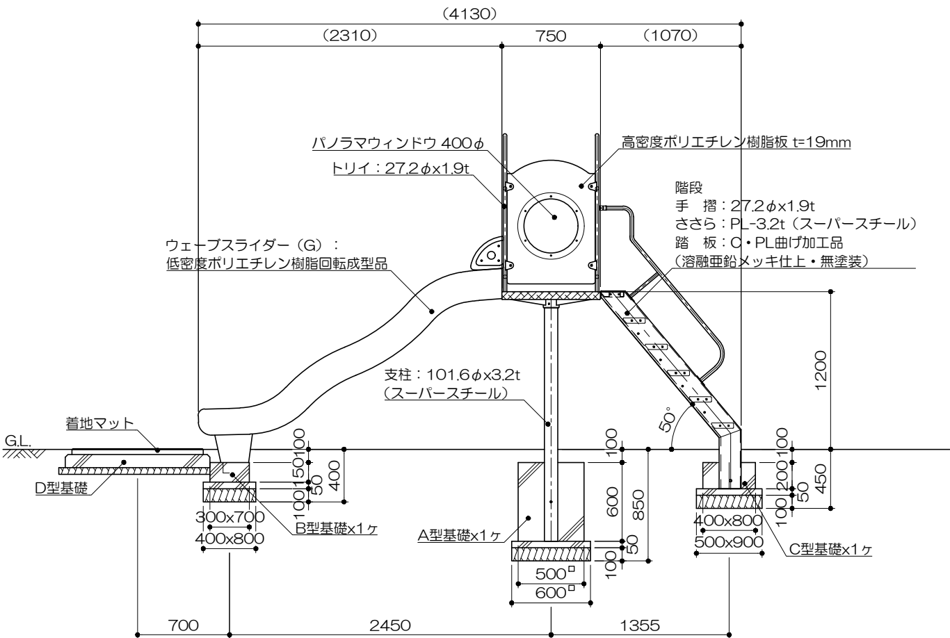
立面図 S= 1 : 40
