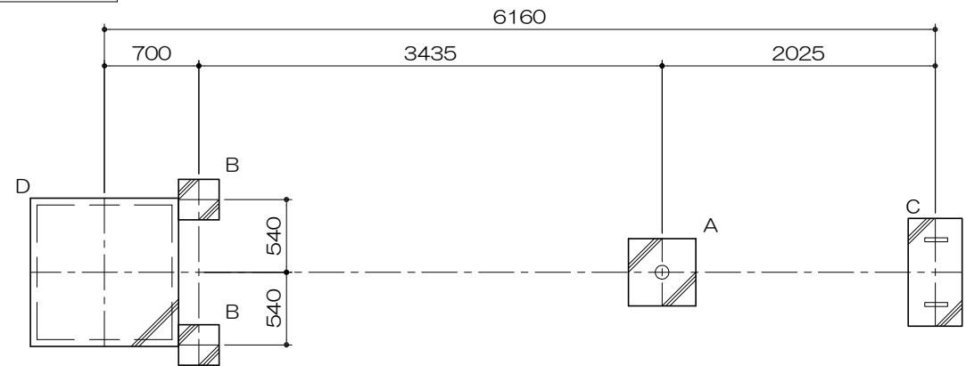
基礎平面図 S= 1 : 50
