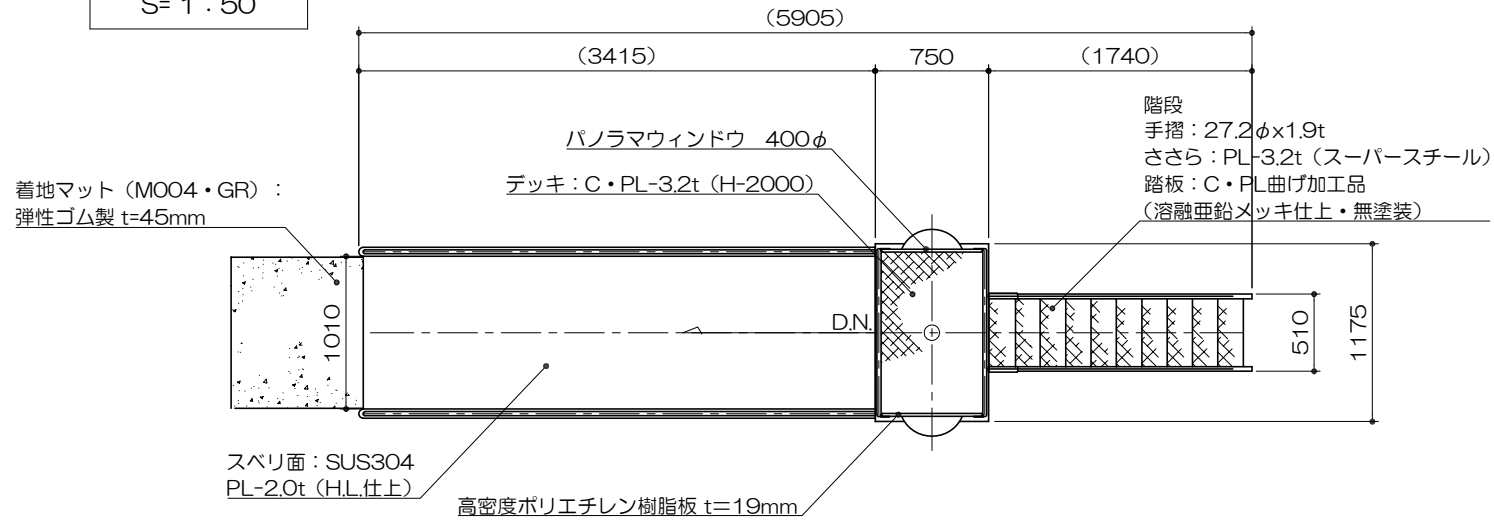
平面図 S= 1 : 50
