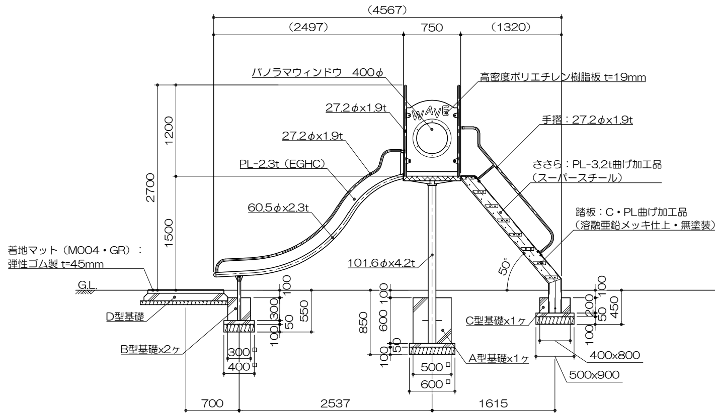
立面図 S= 1 : 50
