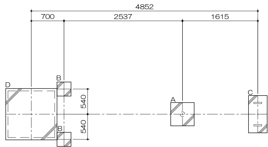
基礎平面図 S= 1 : 50
