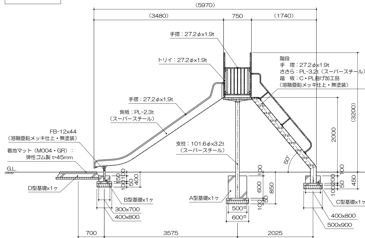
立面図 S= 1 : 50
