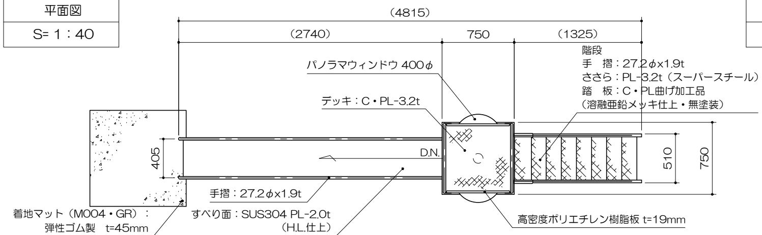
基礎平面図
