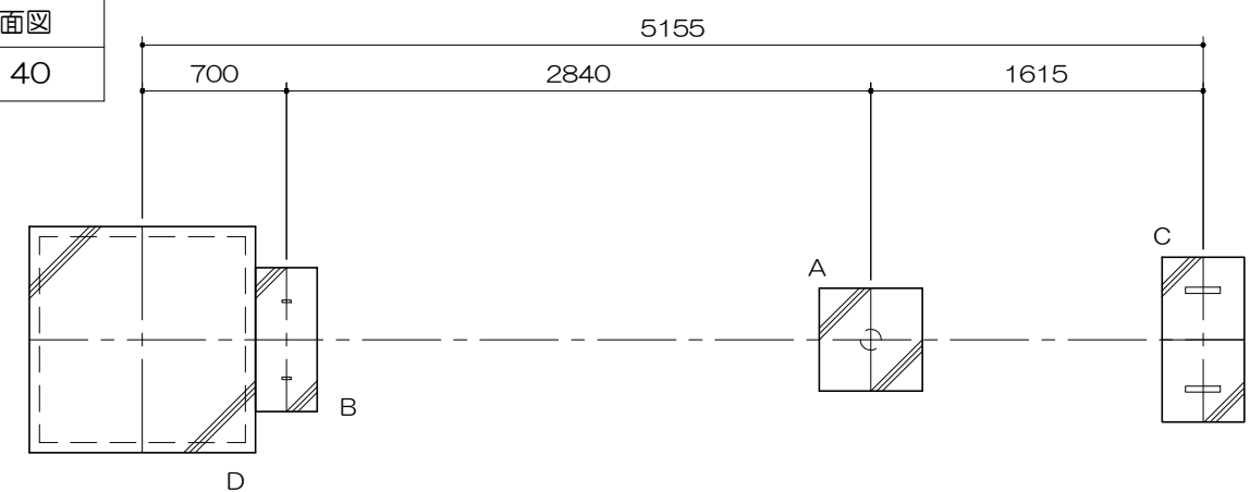
D型基礎詳細図
