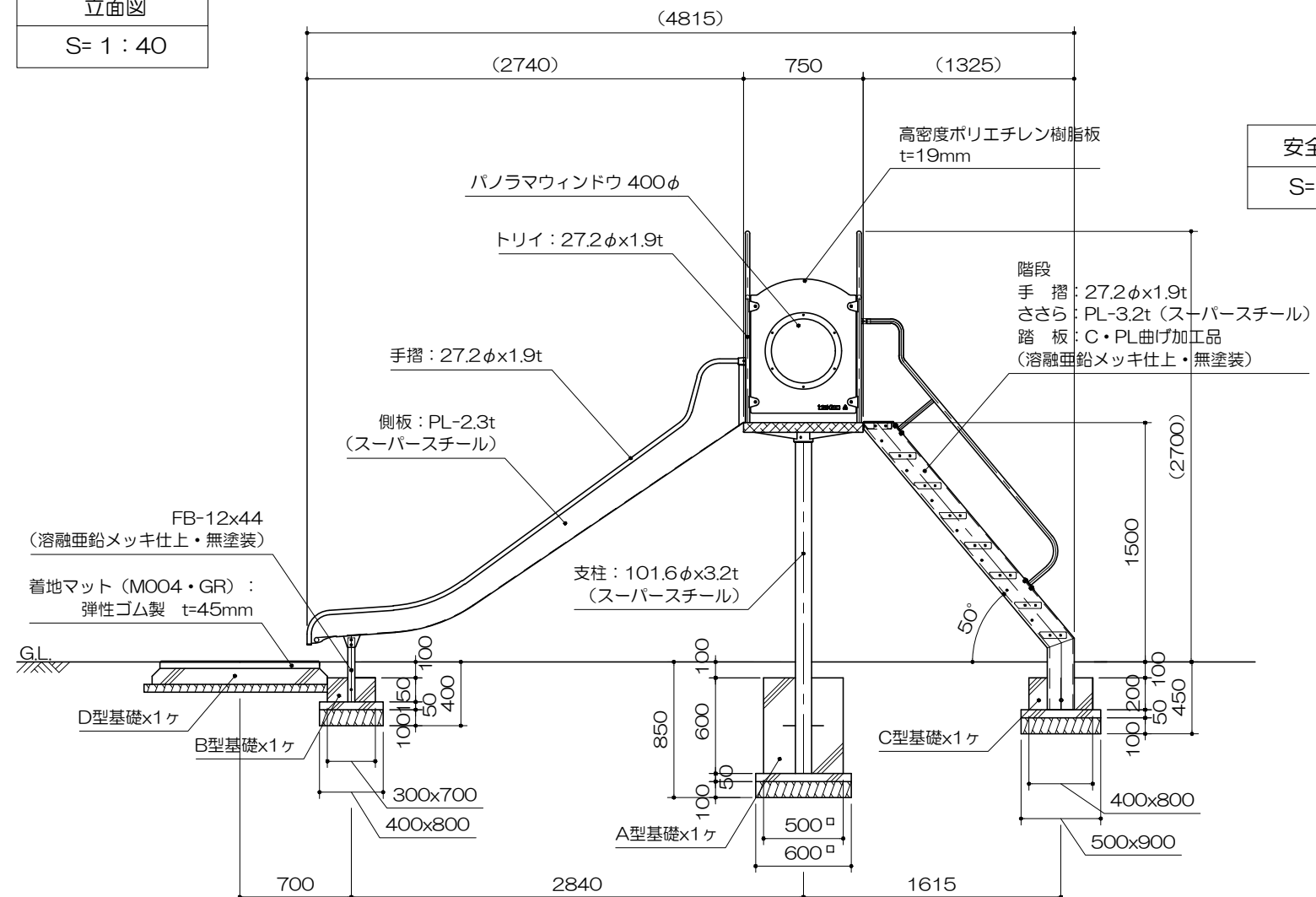
立面图
