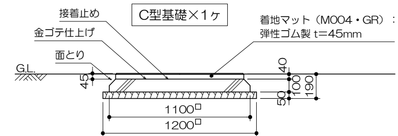
C型基礎詳細図
