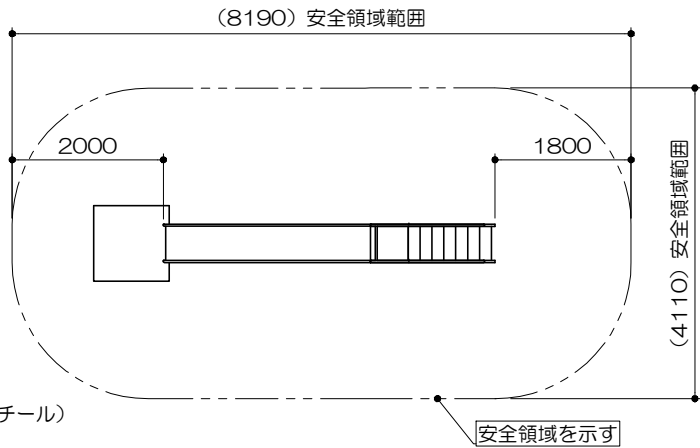
PG33-SU002+マット付 アームスライダー S=図示 (K)
