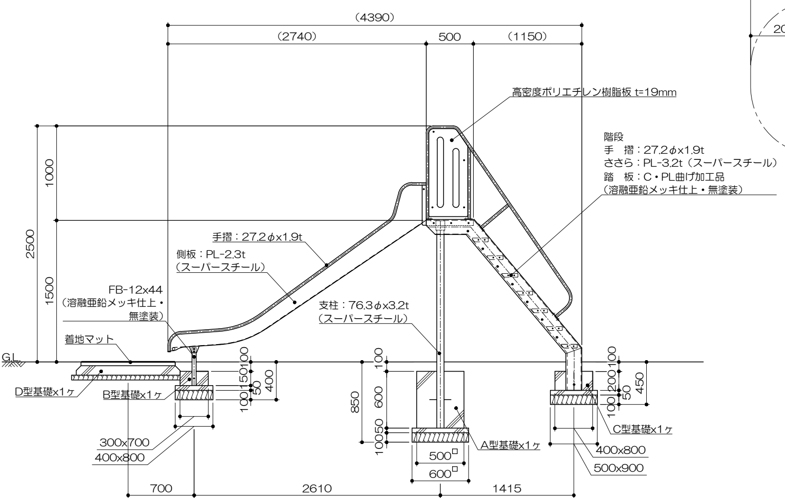
立面図 S= 1 : 40
