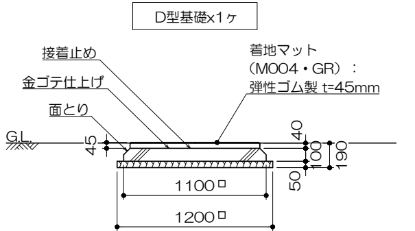
D型基礎詳細図 S= 1 : 40
