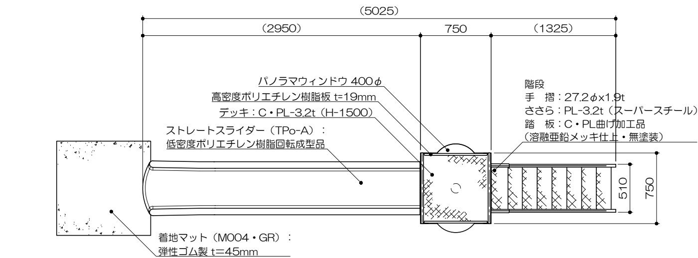
平面図 S= 1 : 40
