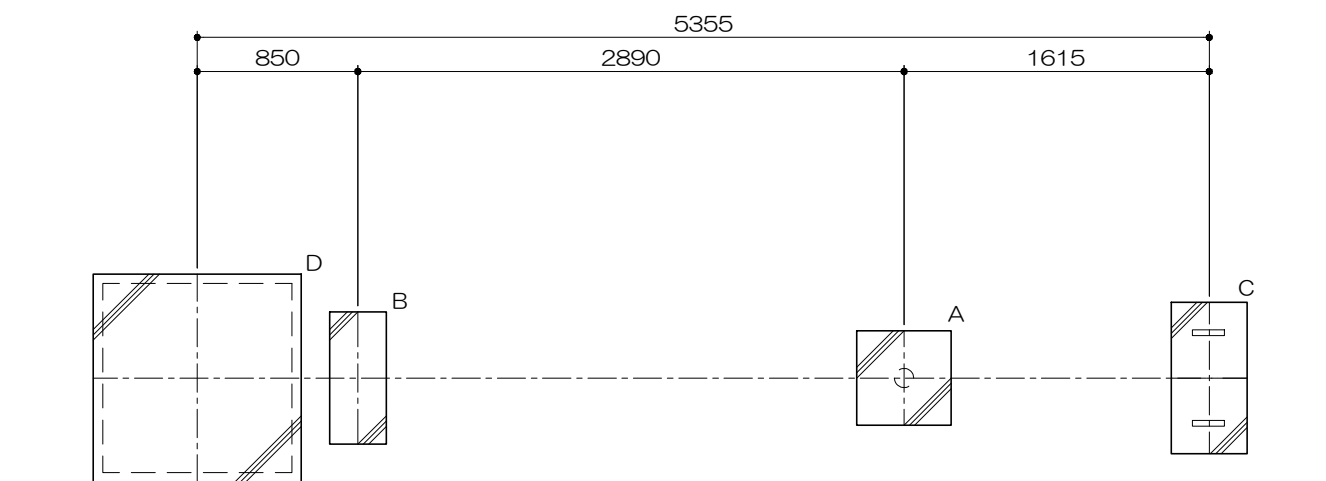
基礎平面図 S= 1 : 40
