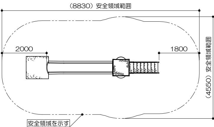
PG33-SU001+マット付 オープンスライダー (H-1500) S=図示 (EK)
