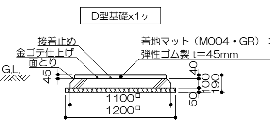
D型基礎詳細図 S= 1 : 40
