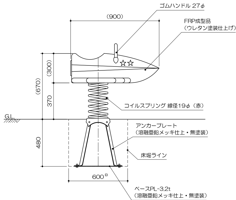
立面図 S= 1 : 20
