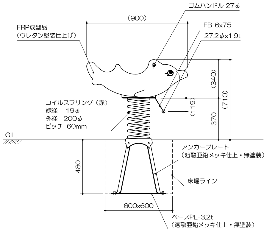
立面図 S= 1 : 20
