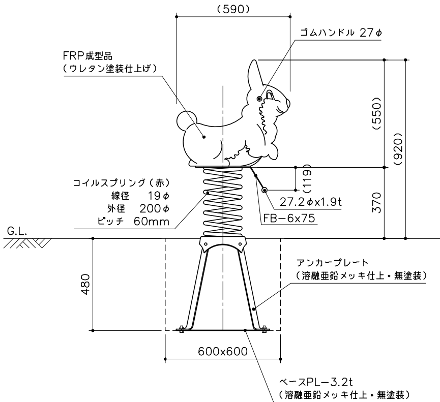
立面図 S= 1:20
