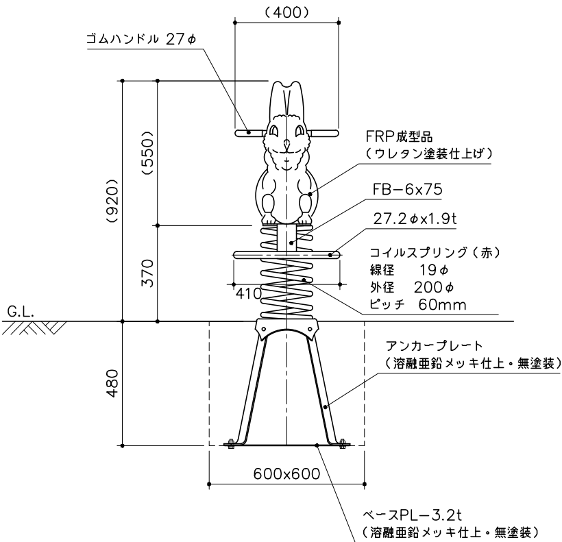
側面図 S= 1:20
