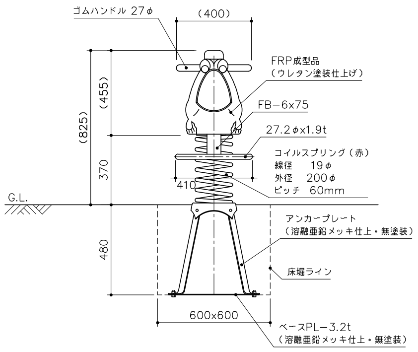
側面図 S= 1:20
