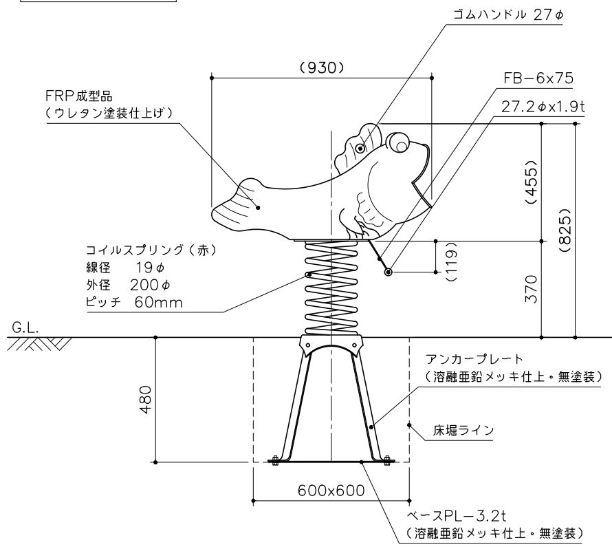
立面図 S= 1:20
