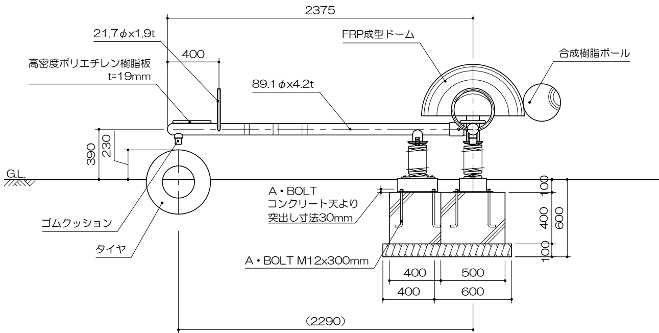
立面図 S= 1 : 30
