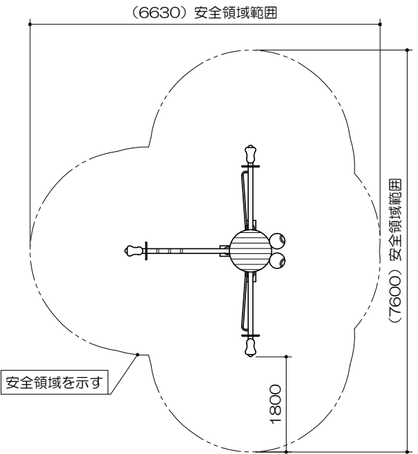
安全領域範囲 S= 1 : 100
