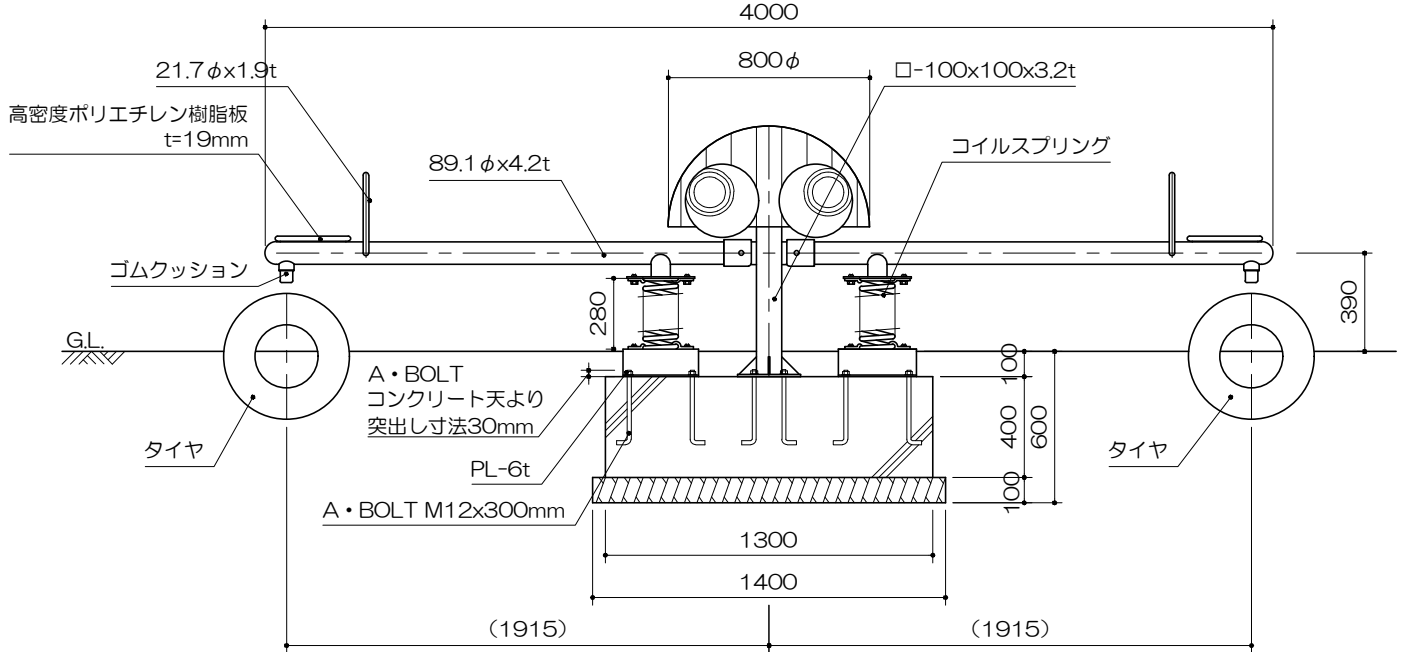
側面図 S= 1 : 30
