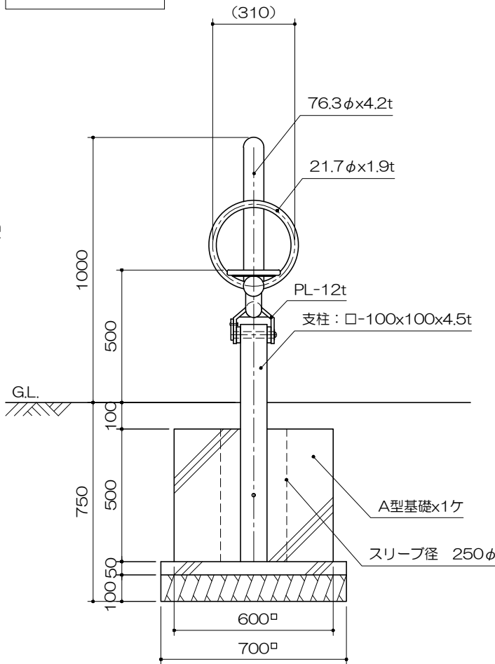
側面図 S= 1 : 20
