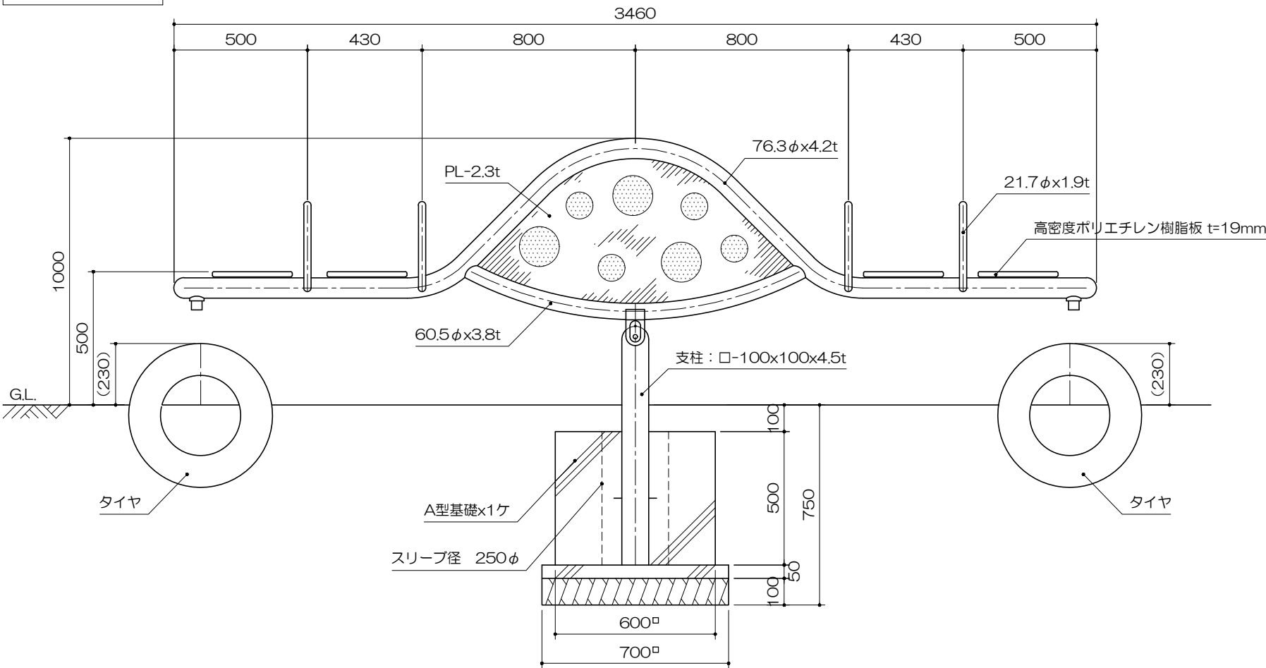
立面図 S= 1 : 20
