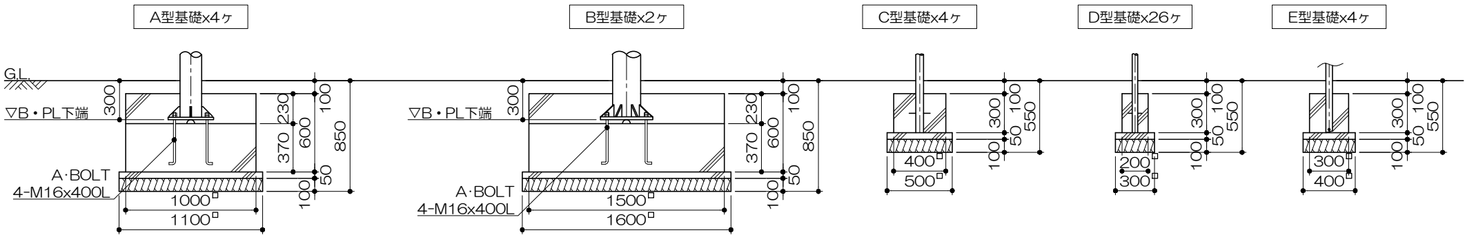
アンカープラン S= 1 : 20
