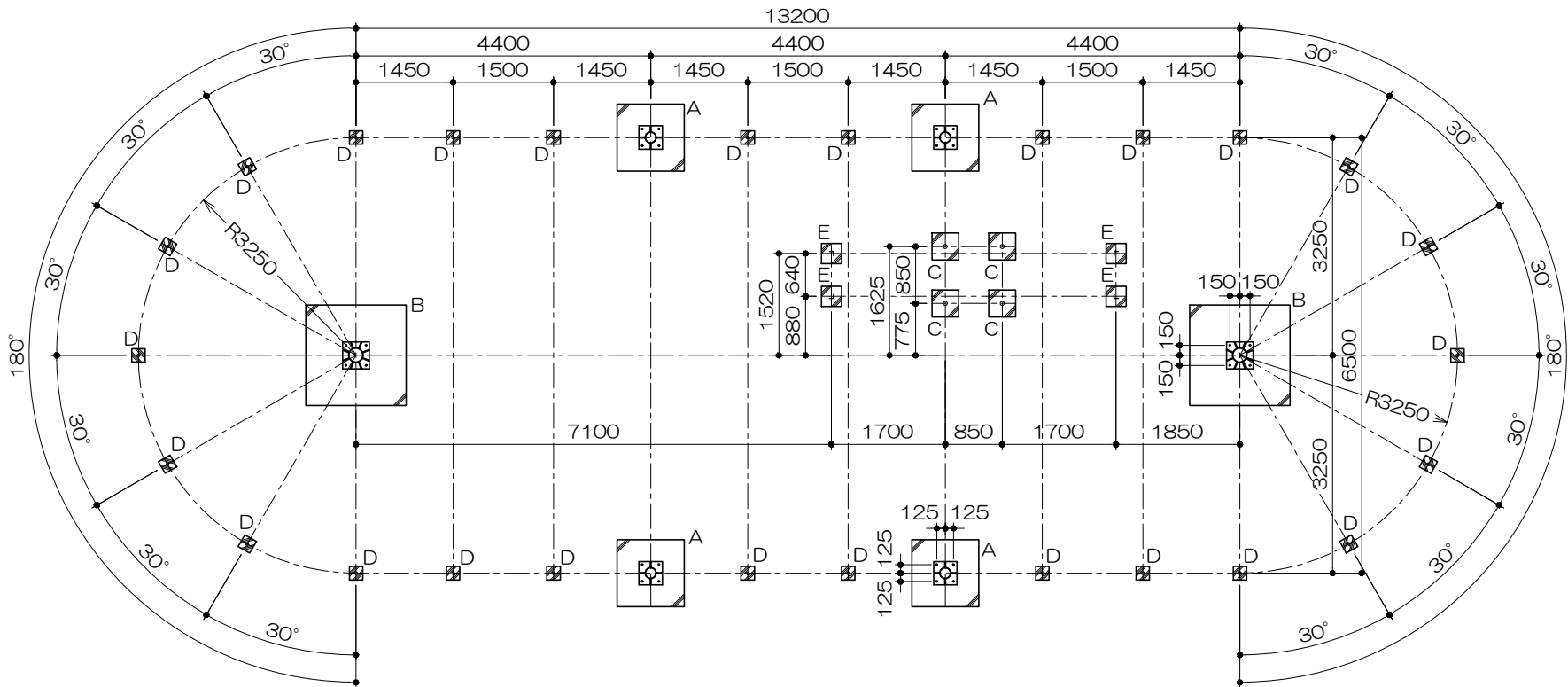
基礎平面図 S= 1 : 100
