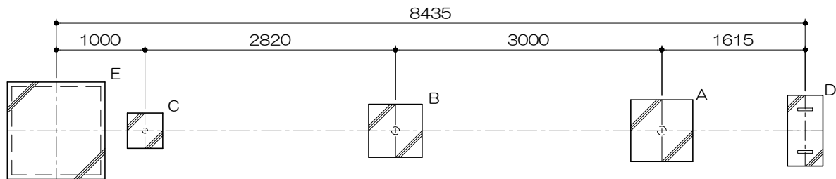
基礎平面図 S= 1 : 60
