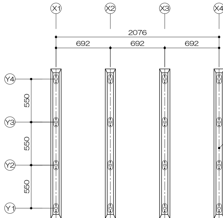
レール平面図 S= 1 : 30
