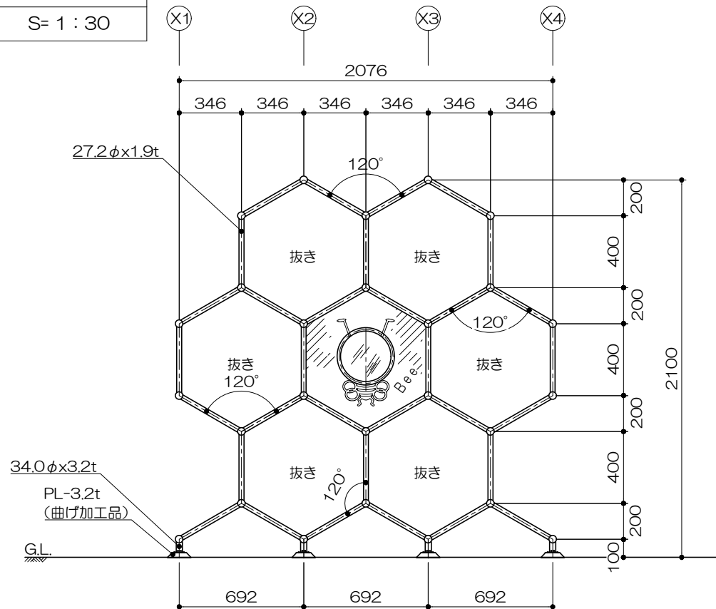
側面図 S= 1 : 30
