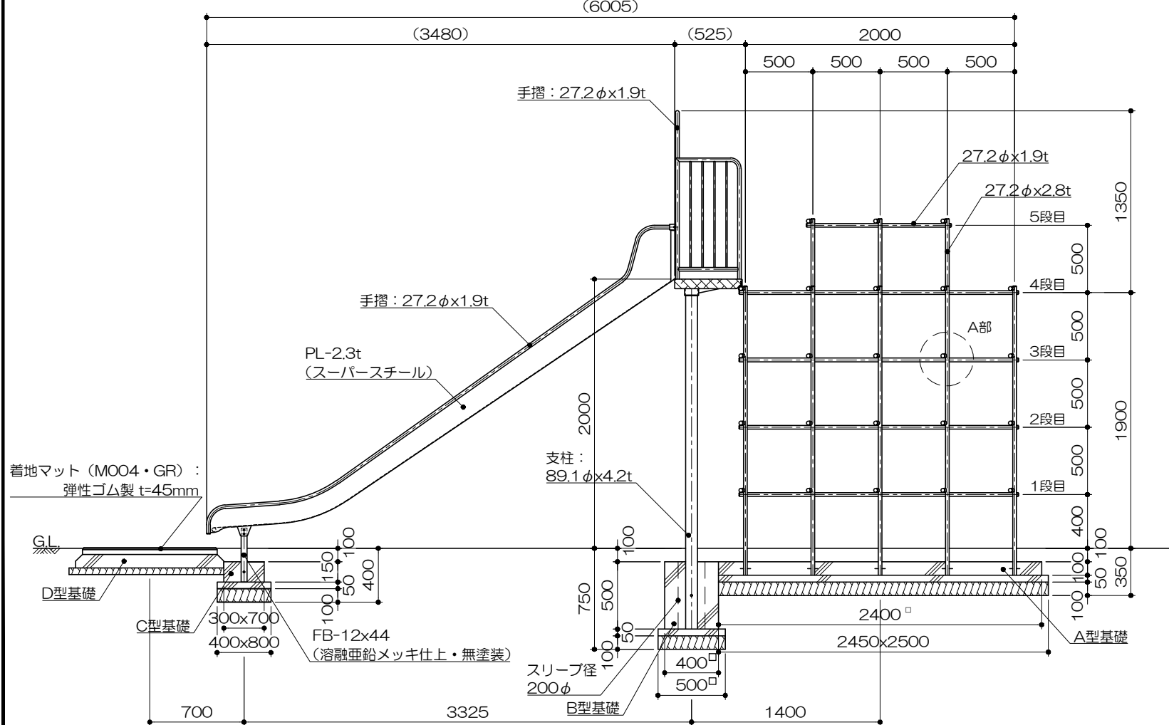
立面図 S= 1 : 40
