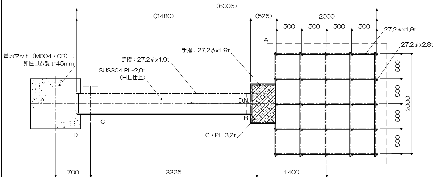
平面図 S= 1 : 40
