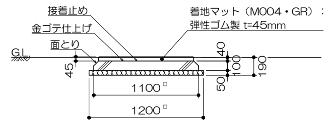
D型基礎詳細図 S= 1 : 40
