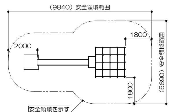
安全領域範囲 S= 1 : 150
