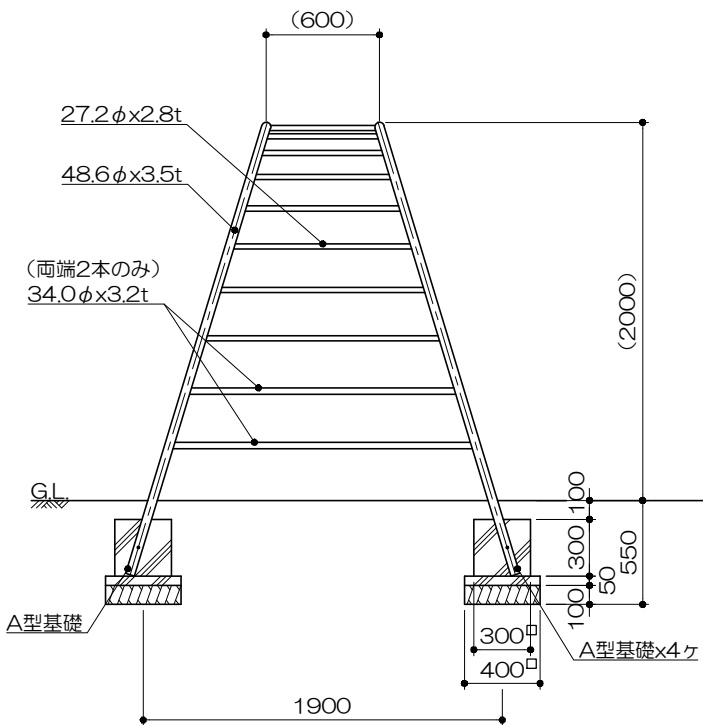
側面図 S= 1：40
