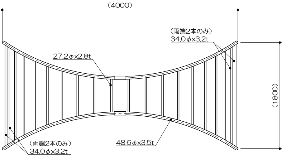
平面図 S= 1：40
