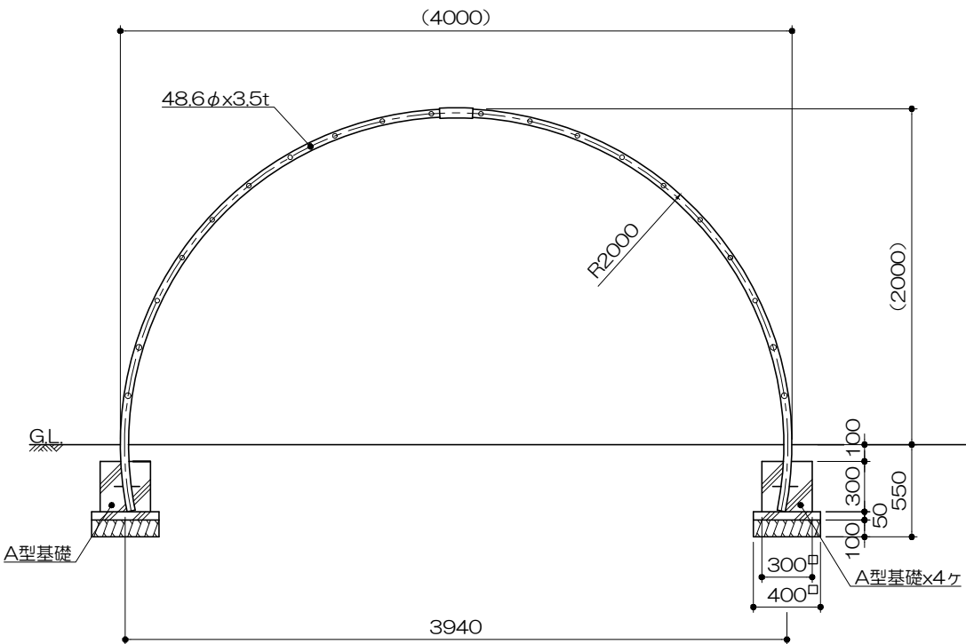
立面図 S= 1：40
