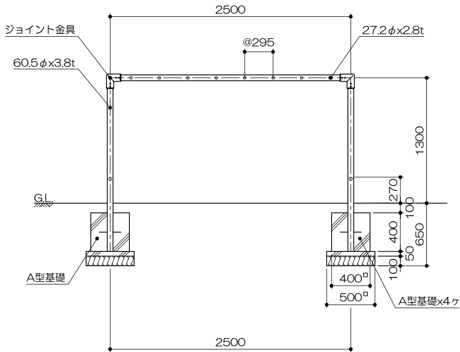
立面図 S= 1 : 40
