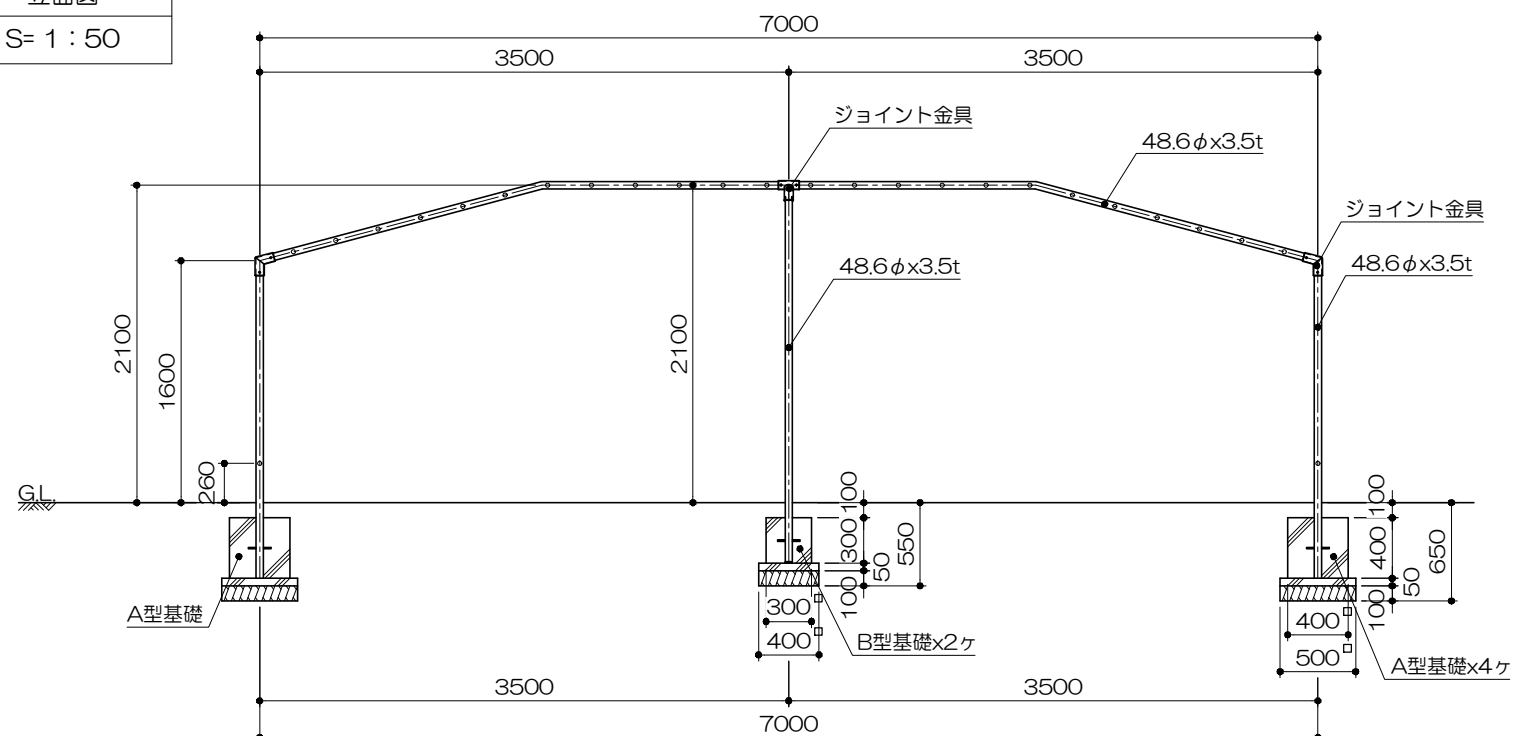
立面图
