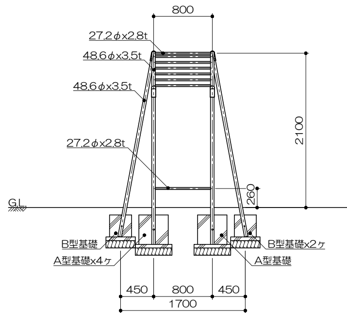
側面図 S= 1 : 50
