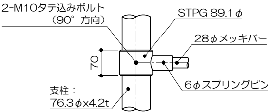
う部詳細図 S= 1 : 10
