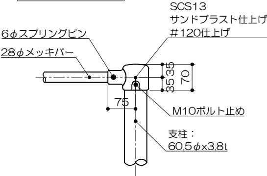
え部詳細図 S= 1 : 10
