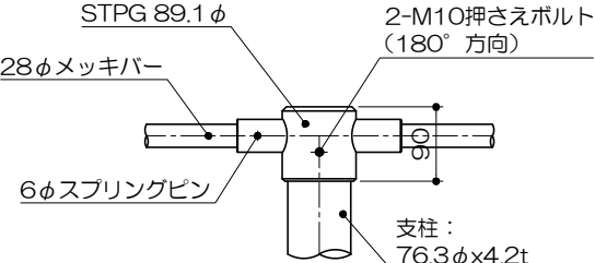
え部詳細図 S= 1 : 10
