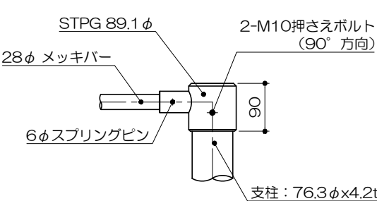
え部詳細図 S= 1 : 10
