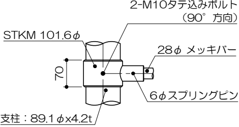
う部詳細図 S= 1 : 10
