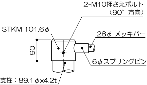
あ部詳細図 S= 1 : 10
