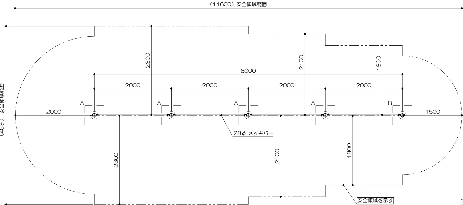
平面図 S= 1 : 50
