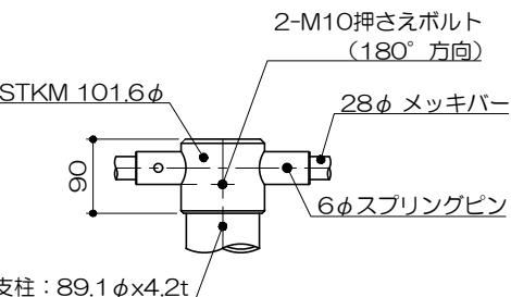
い部詳細図 S= 1 : 10
