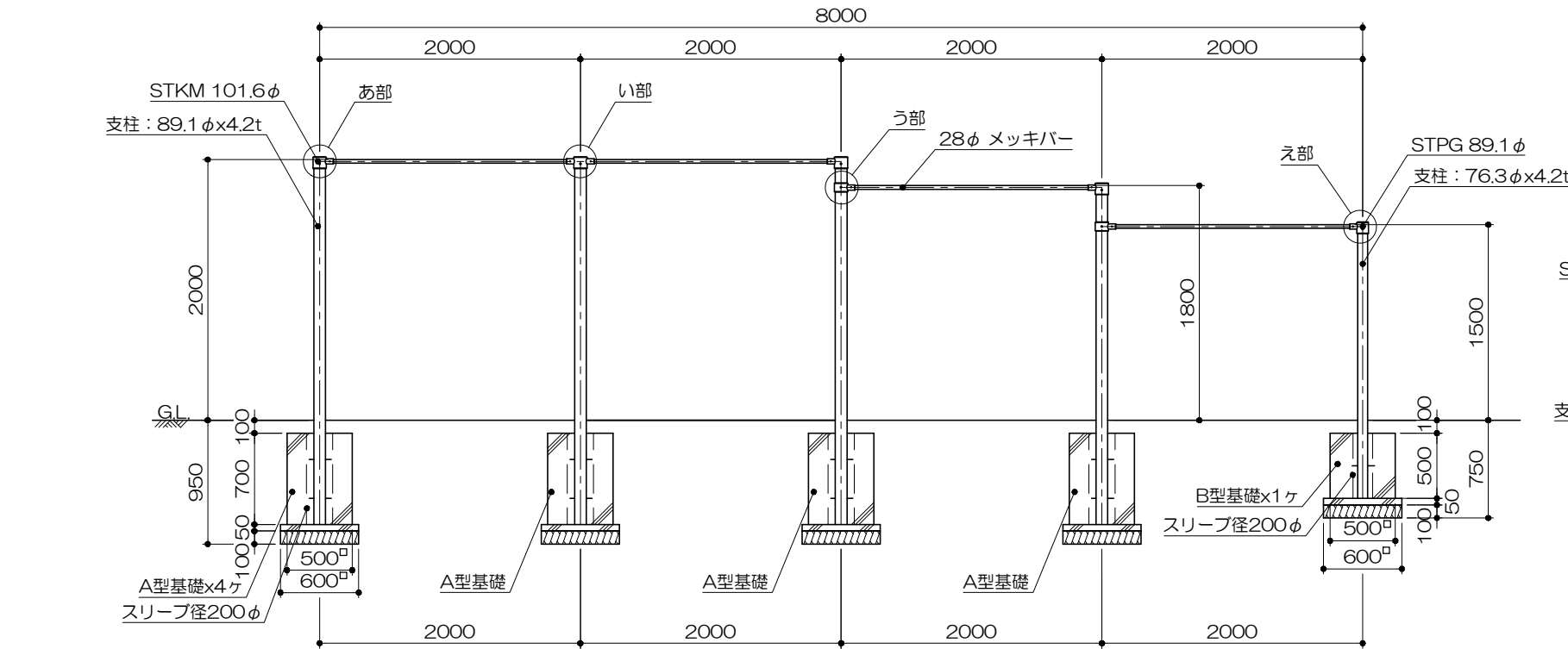
立面図 S= 1 : 50
