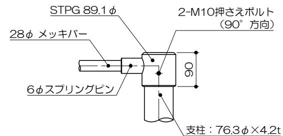
う部詳細図 S= 1 : 10
