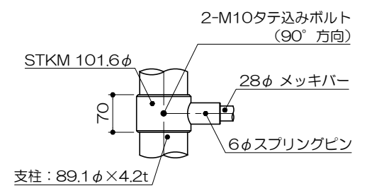
い部詳細図 S= 1 : 10
