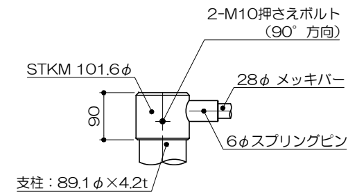
あ部詳細図 S= 1 : 10
