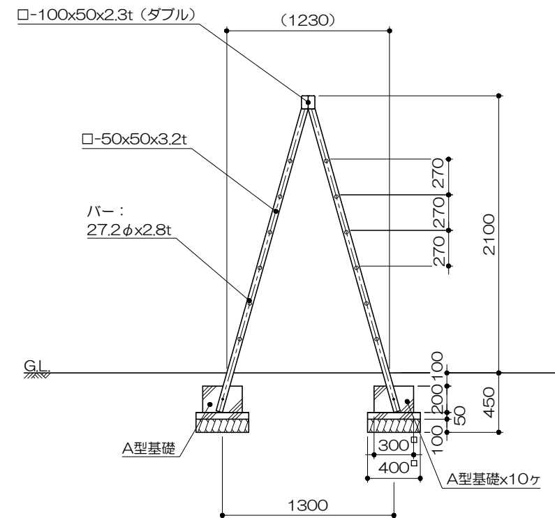
側面図 S= 1 : 40
