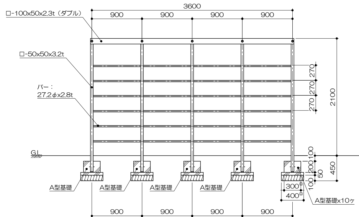
立面図 S= 1 : 40
