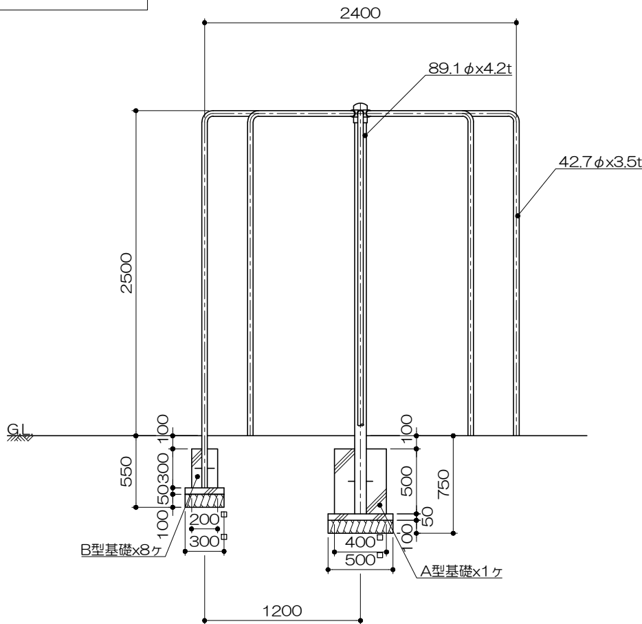
立面図 S= 1 : 40
