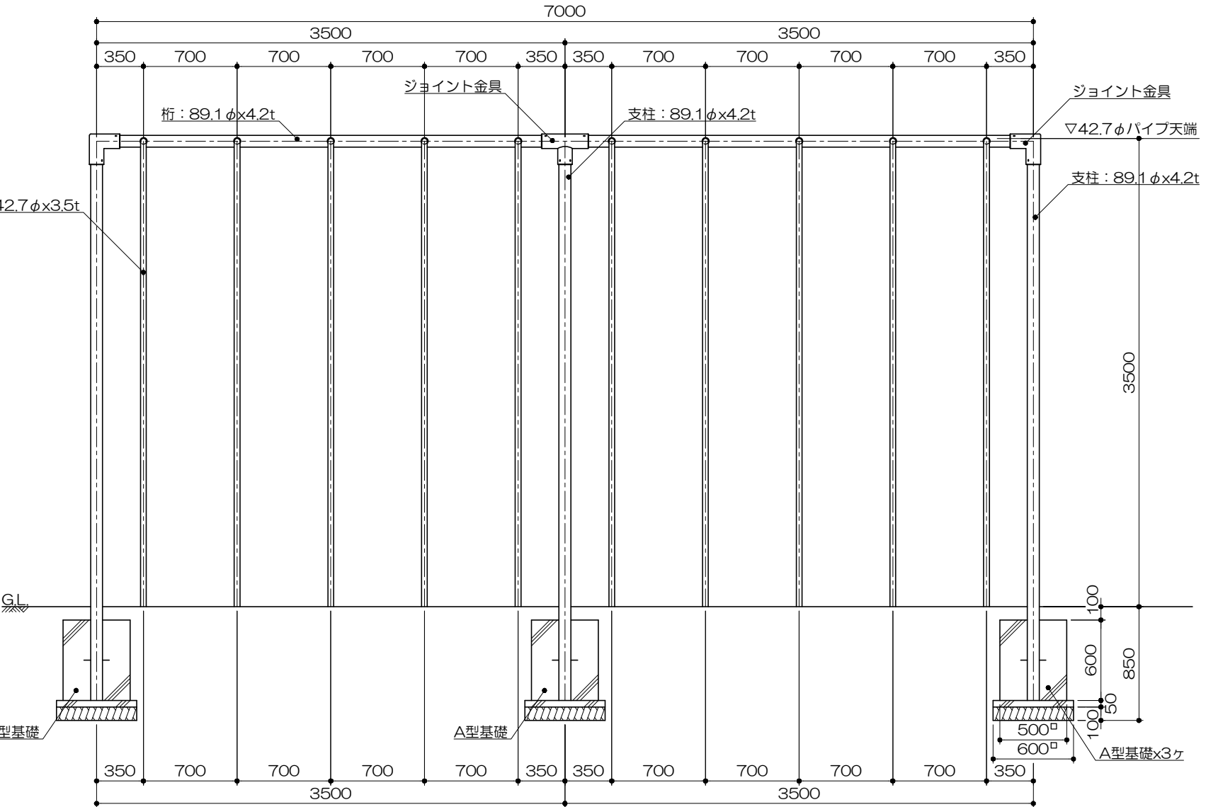
立面図 S= 1 : 40
