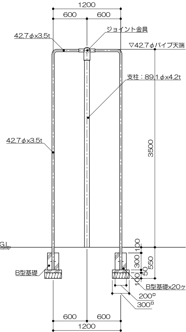
側面図 S= 1 : 40
