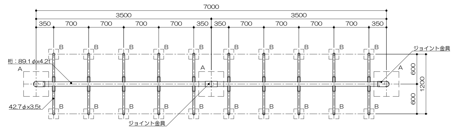
平面図 S= 1 : 40
