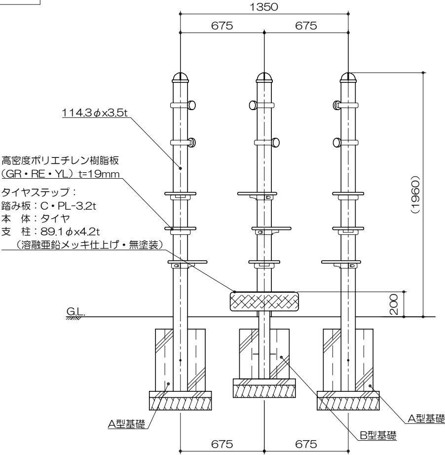
立面図 S= 1 : 30
