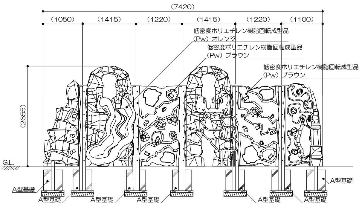
立面図 S= 1 : 60
