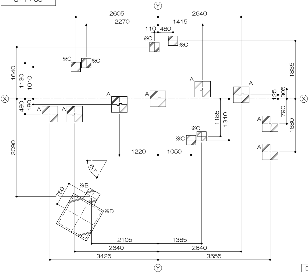
PG33-CL008+マット付 ロックブロック (5) S=図示 (KE)
