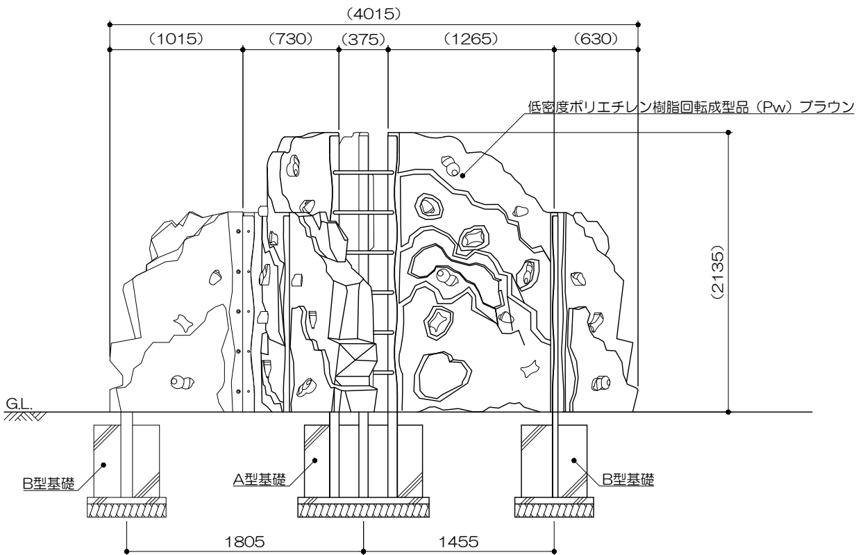
立面図 S= 1 : 40
