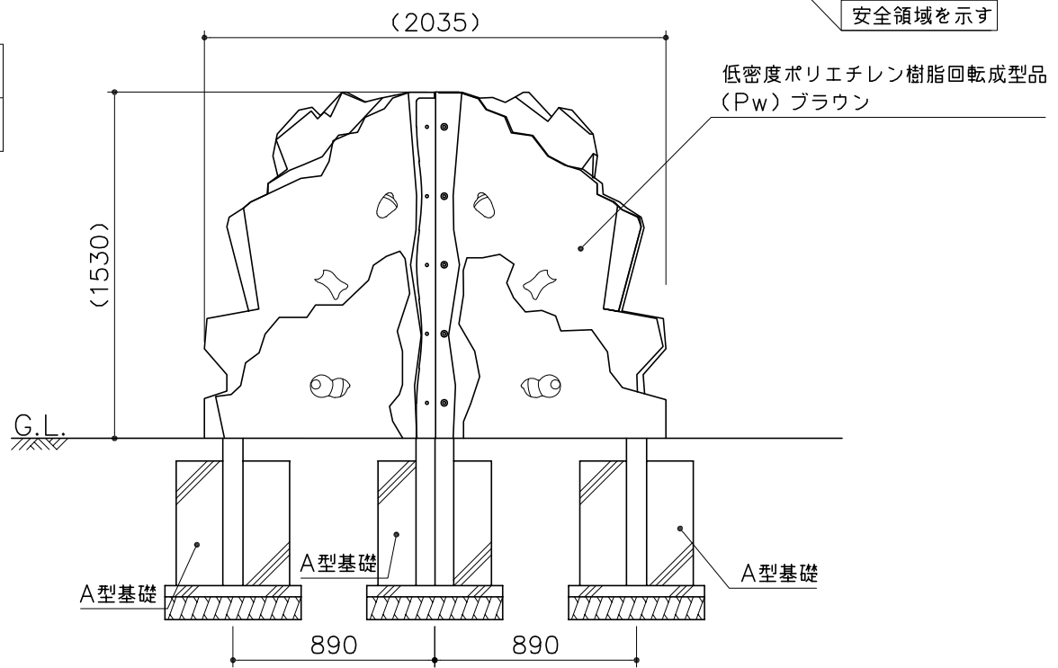
立面図 S= 1 : 30
