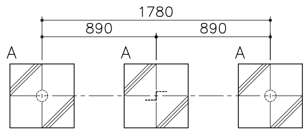
基礎平面図 S= 1 : 30
