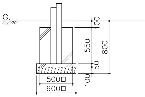
A型基礎×3ヶ
