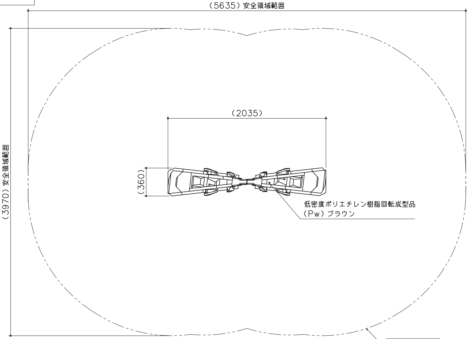
平面図 S= 1 : 30
